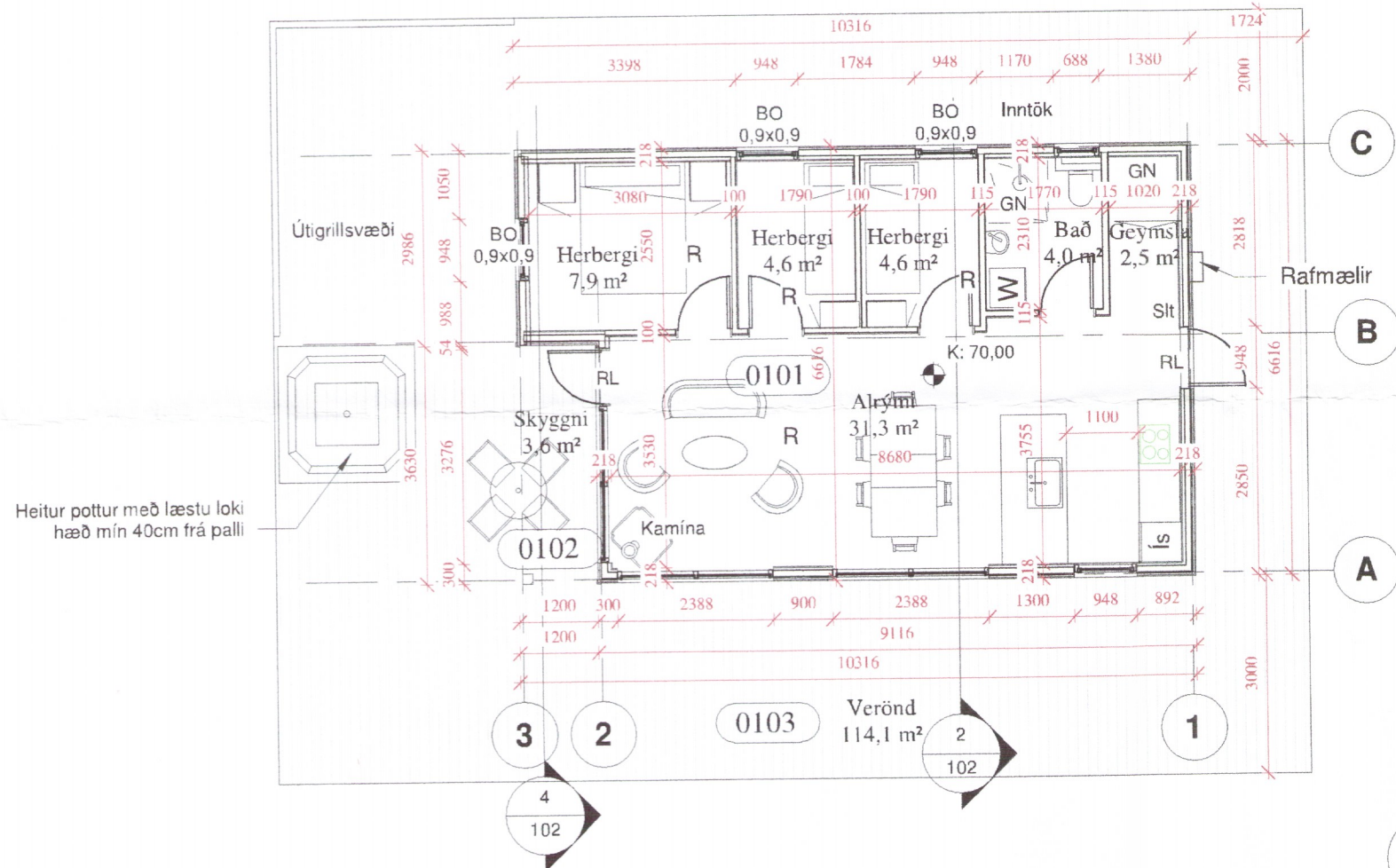
1 GRUNNMYND 1 : 100
