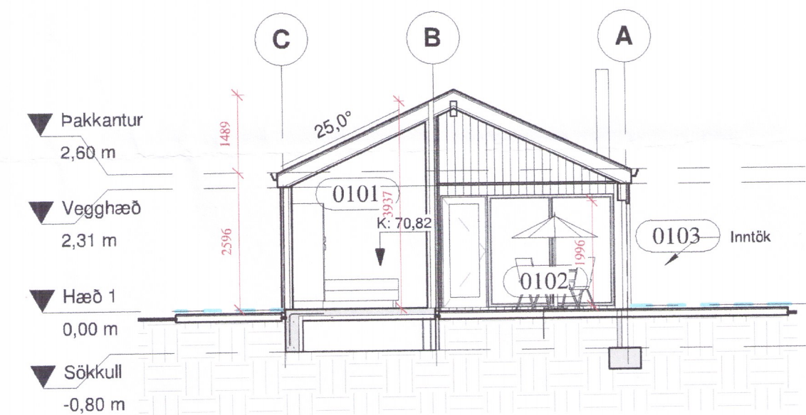
4 PVERSKURÐUR VIÐ ANDDYRRI 1 : 100
