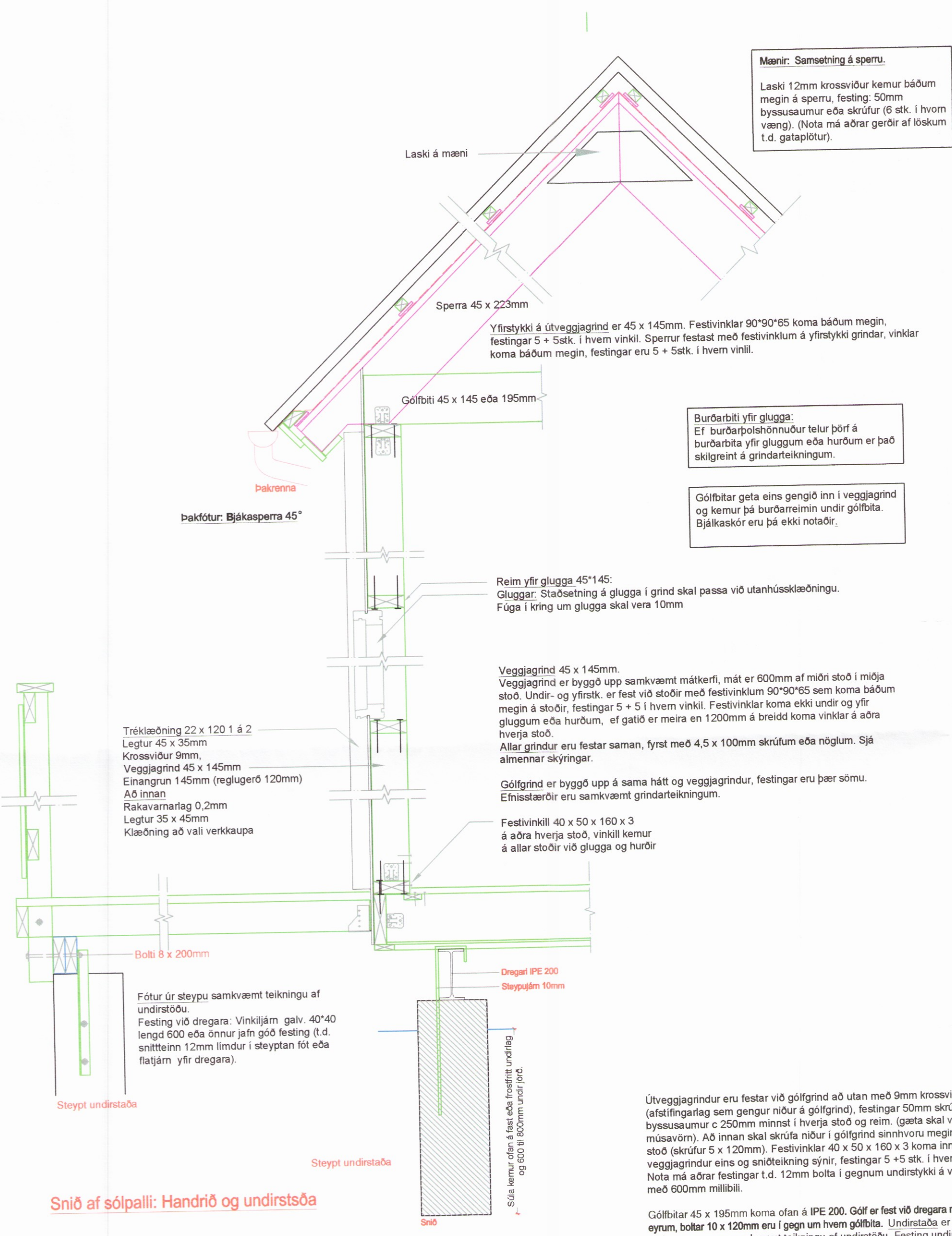
Snið lóðrétt mynd: Útveggur:
