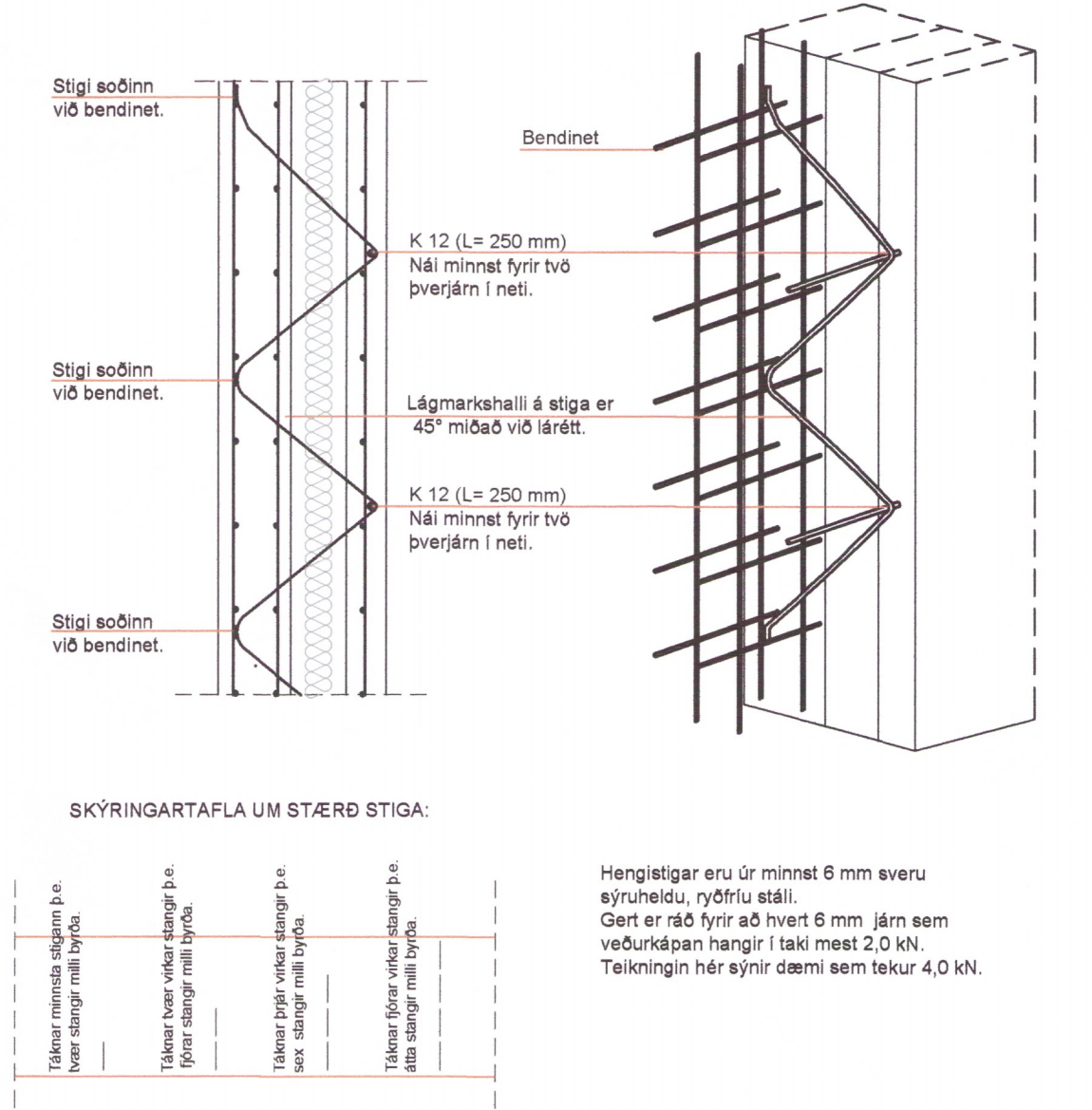
TENING INNRA OG YTRA BYRÐIS Ekki í kvarða
