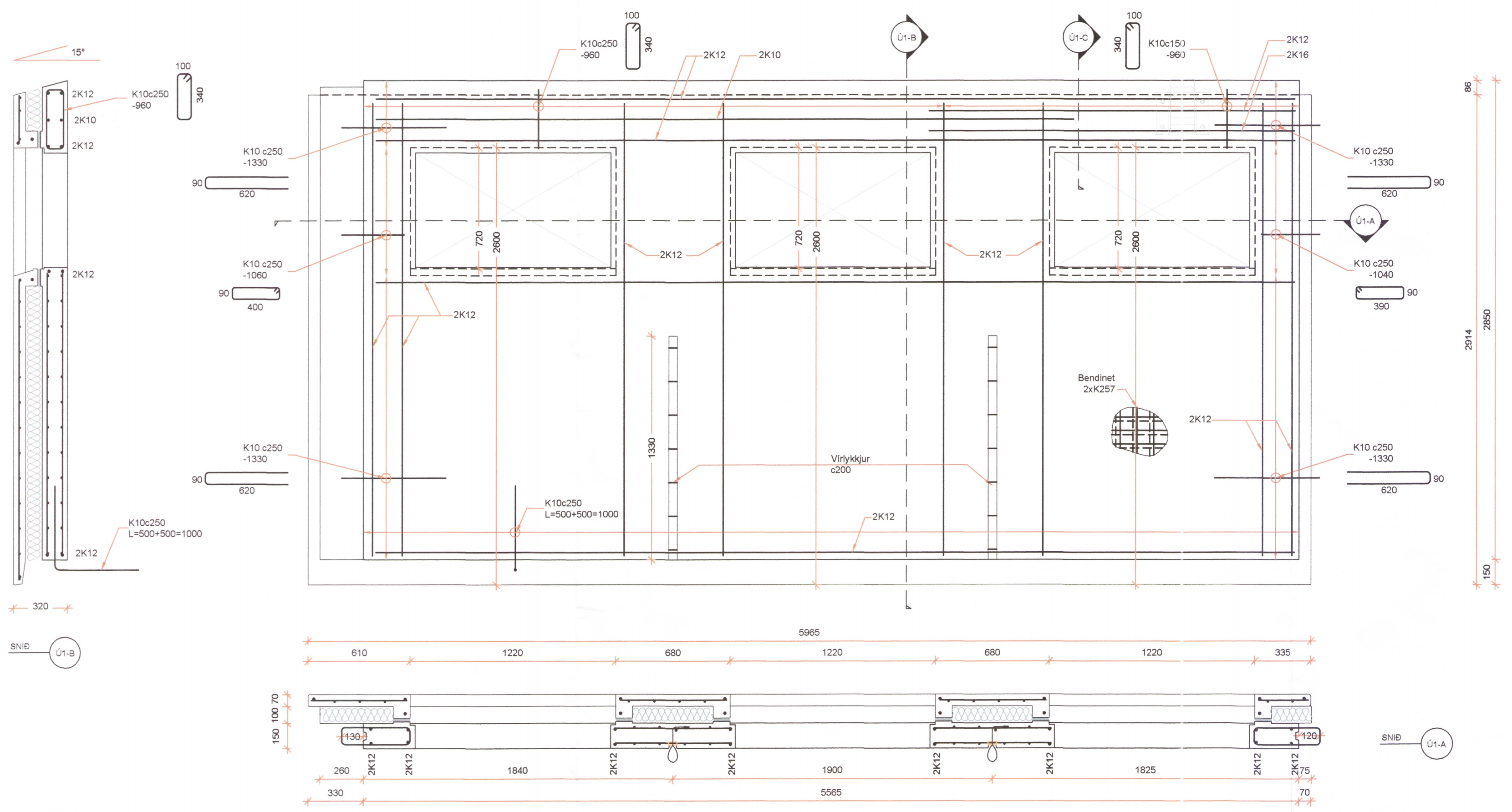
Ú1 - ÚTVEGGJAEINING Mkv. 1:20 ÁSÝND INNANFRÁ
