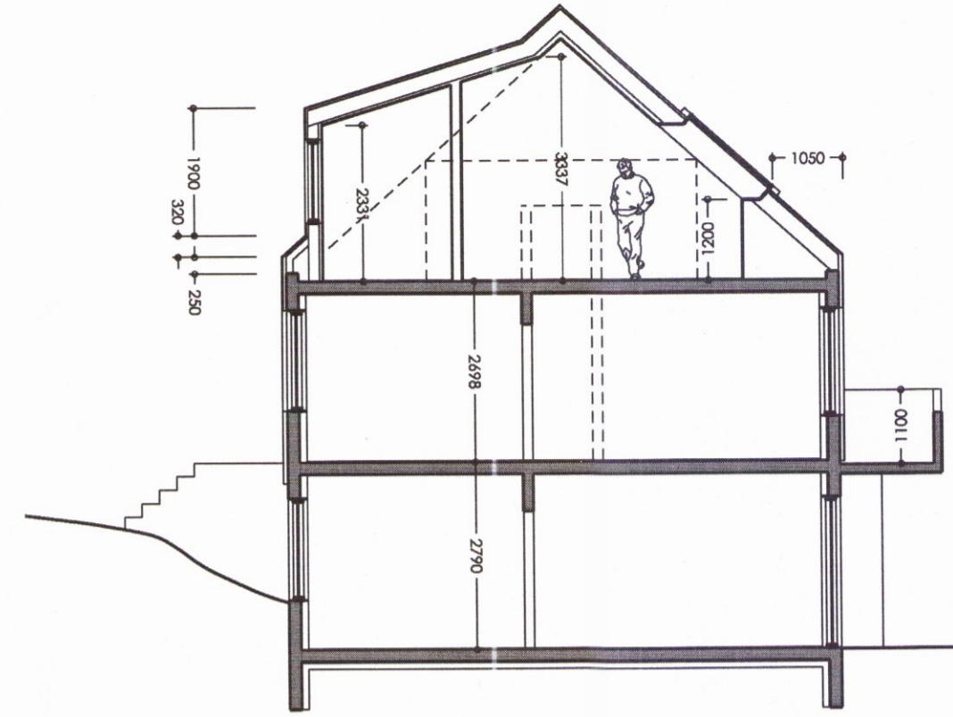
Sneið BB
