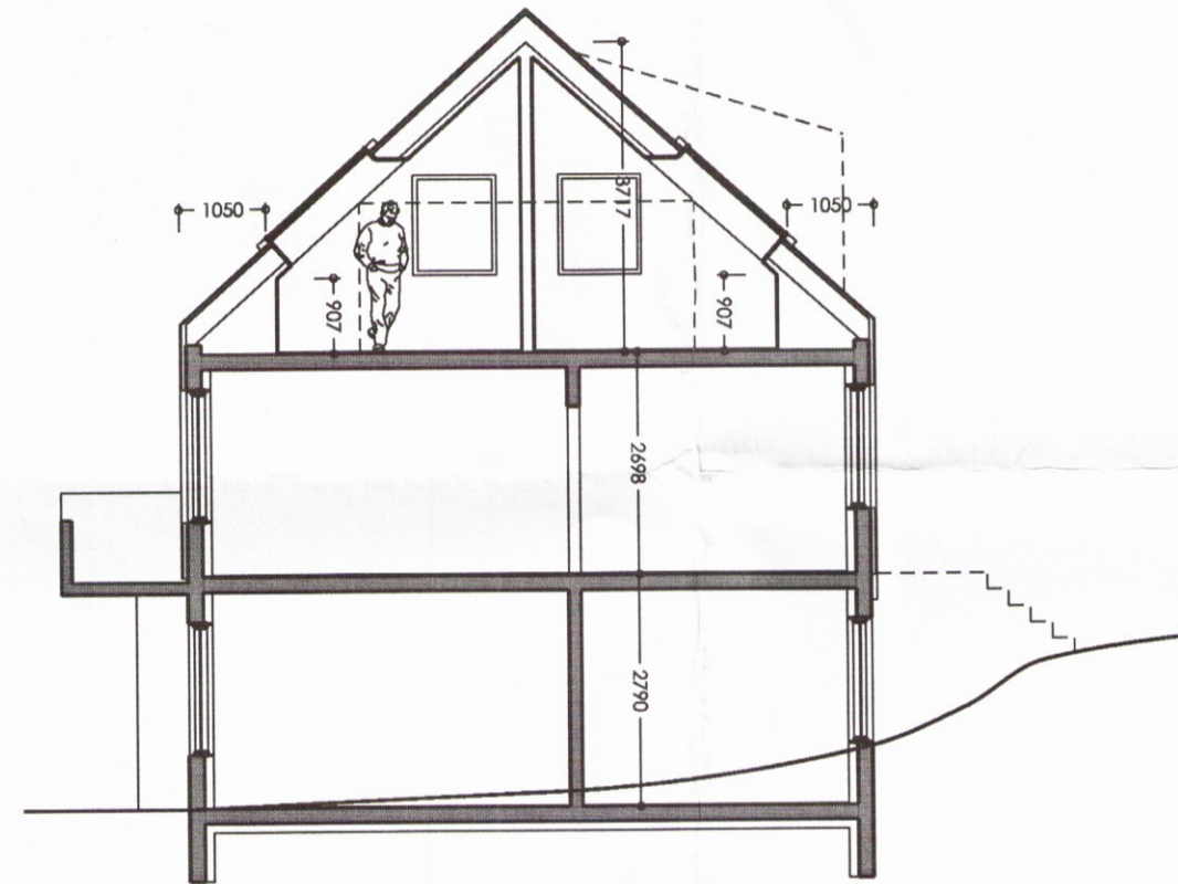
Sneið AA
