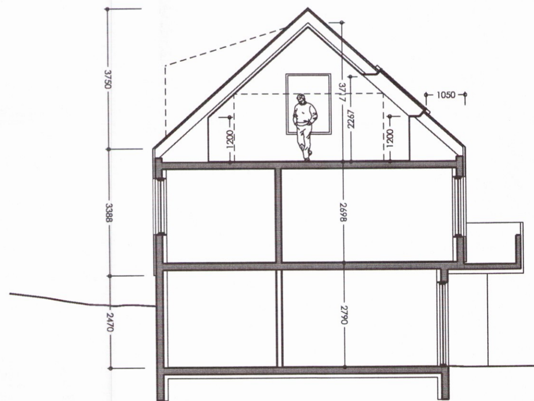
Sneið CC
