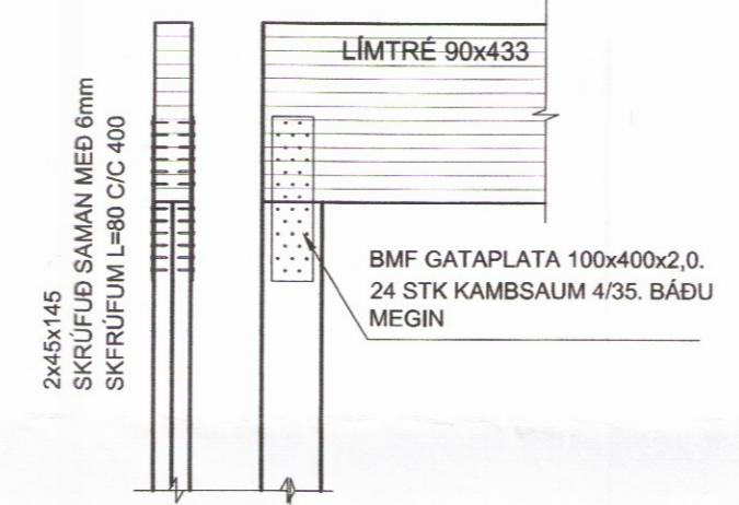
J SNIÐ B4 M. 1: 20
