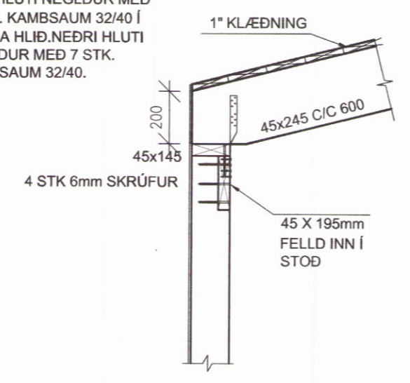
G SNIÐ B4 M. 1: 20
