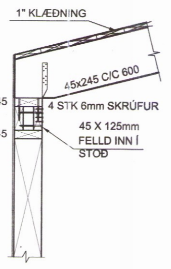
H SNIÐ B4 M. 1: 20
