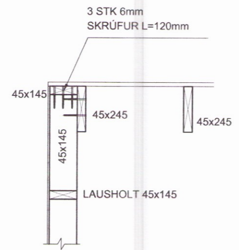
E SNIÐ B4 M. 1: 20
