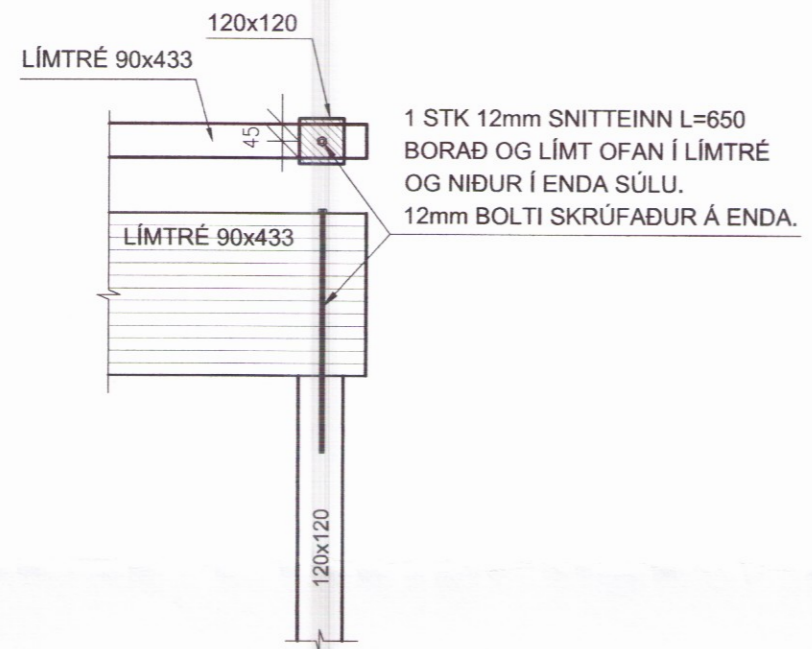
I SNIÐ B4 M. 1: 20
