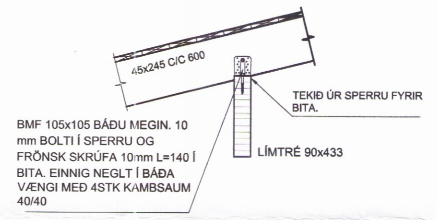
K SNIÐ B4 M. 1: 20
