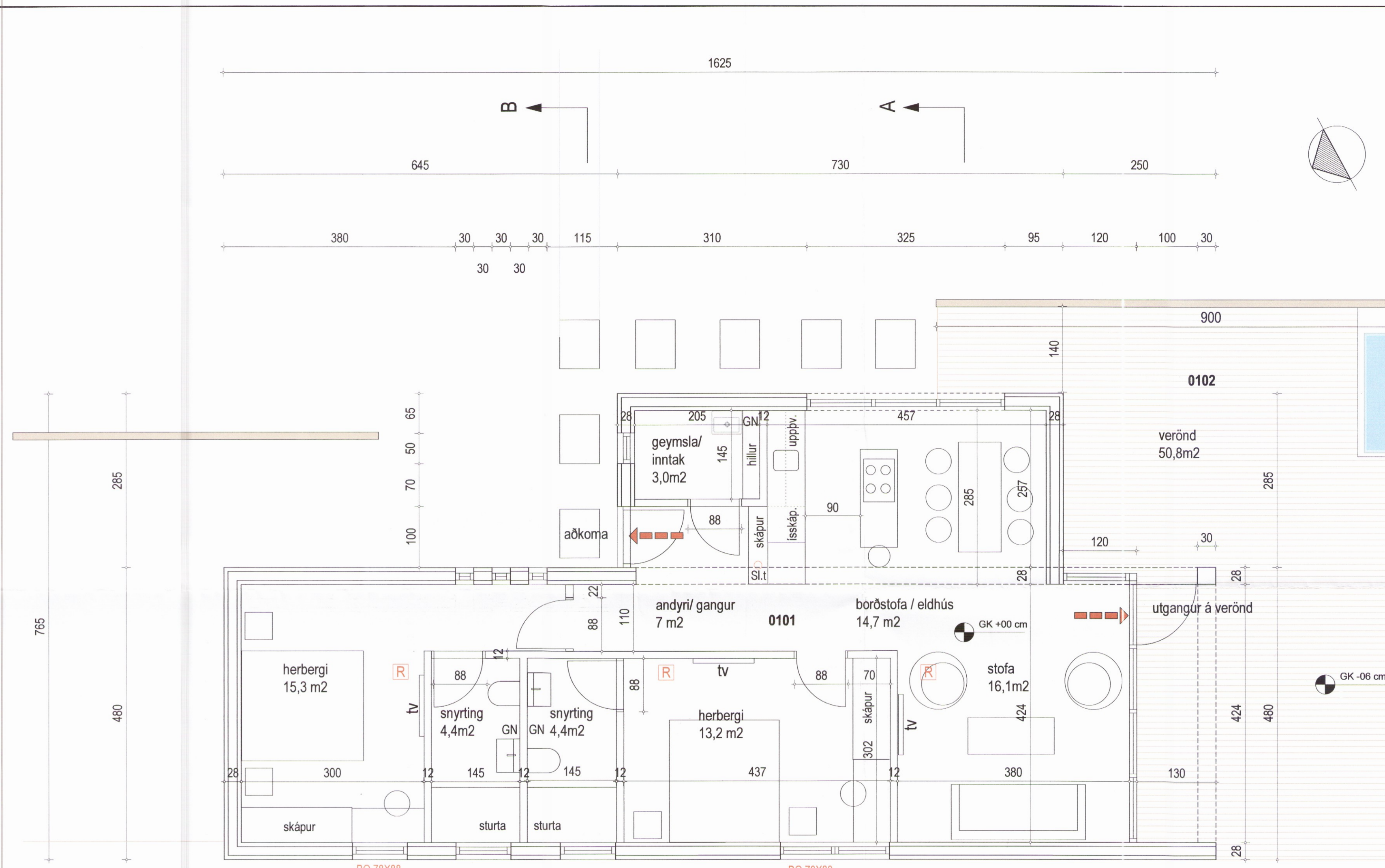
Grunnmynd 1.50
