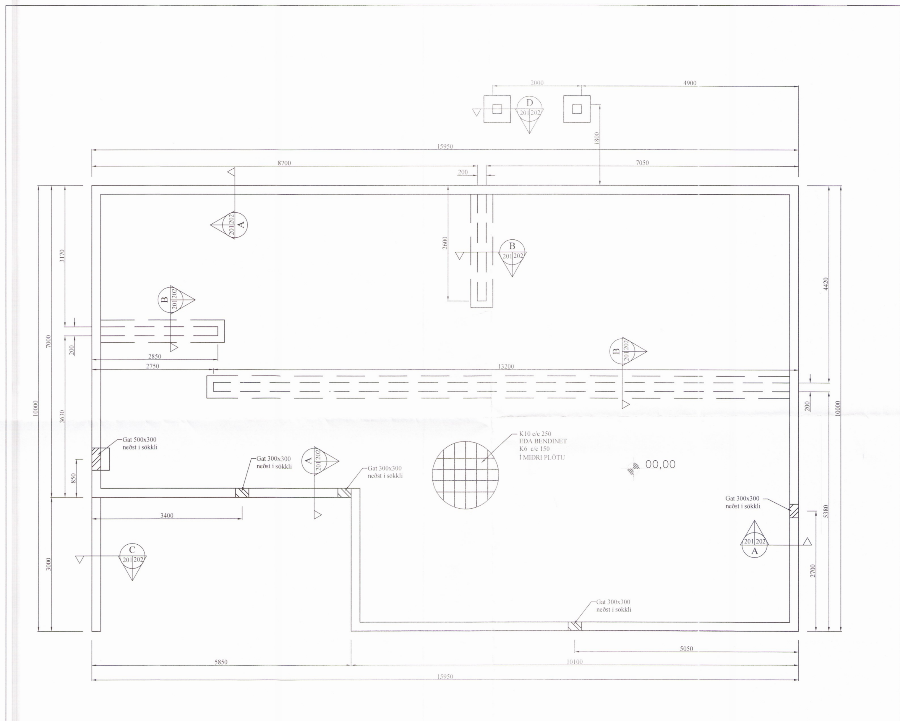
GRUNNMYND SÖKKULS Mkv. 1:50
