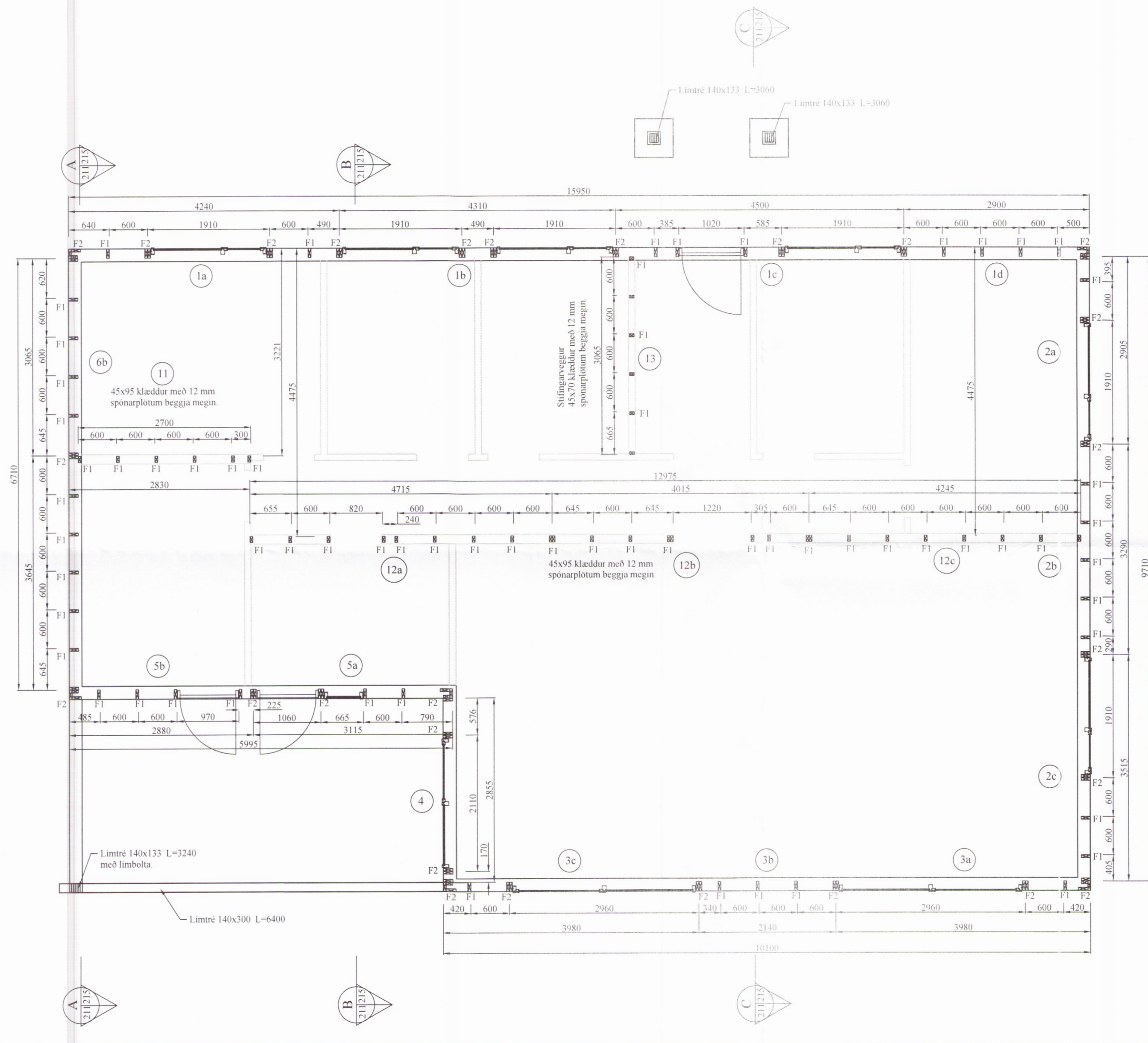
Grunnmynd útveggja MKV. 1:50
