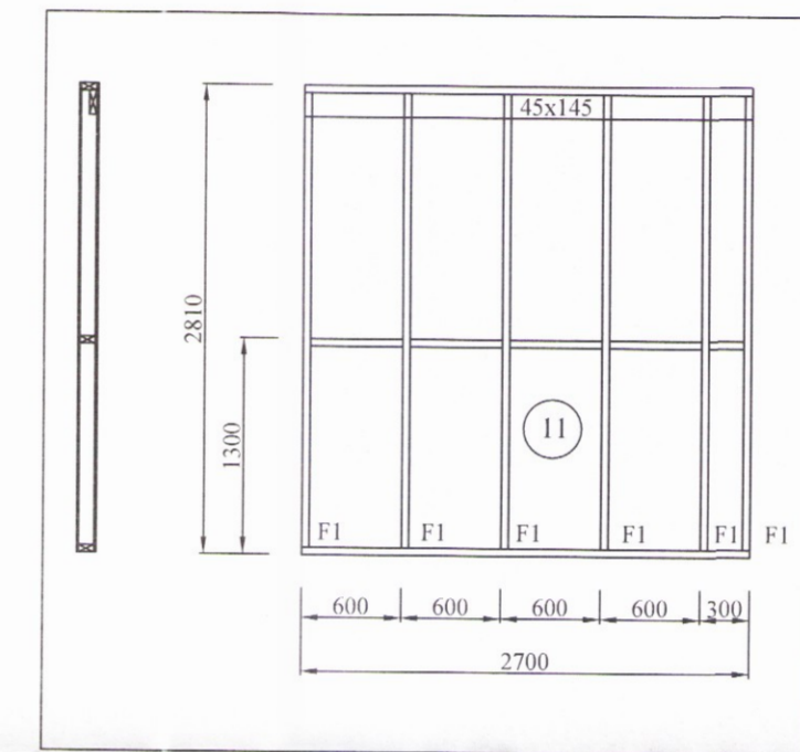
Ásýnd innveggja, burðarveggir og stífingarveggur MKV. 1:50
