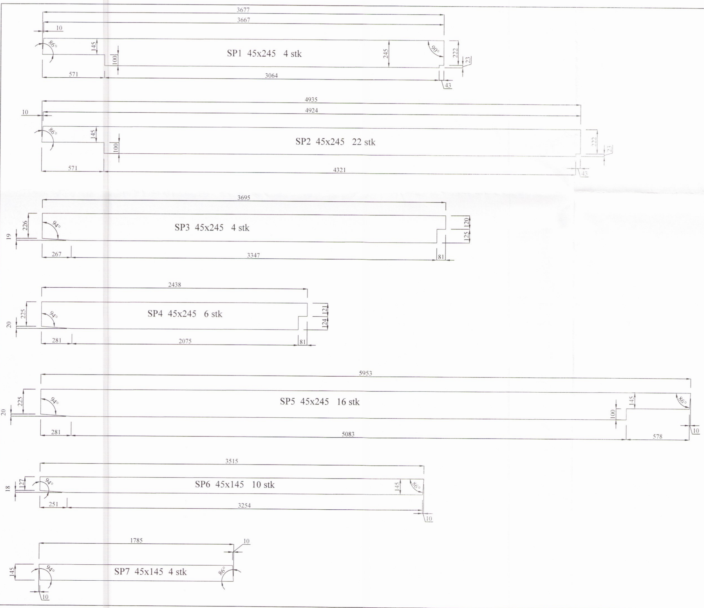
Hliðarmynd sperra MKV. 1:20
