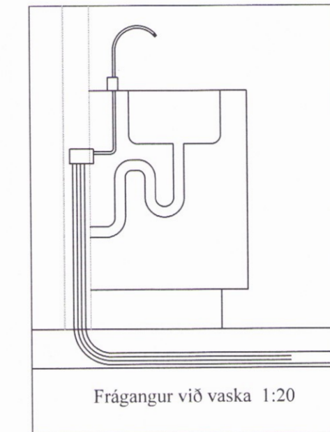
GRUNNMYND VATNSLAGNA Mkv. 1:50
