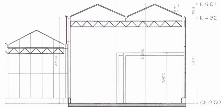
Sníð A-A
