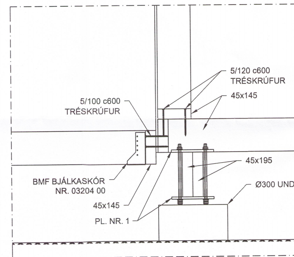
09 DEILI B005 1:10
