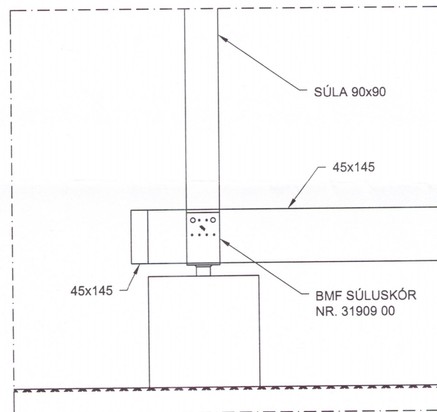
07 DEILI B005 1:10
