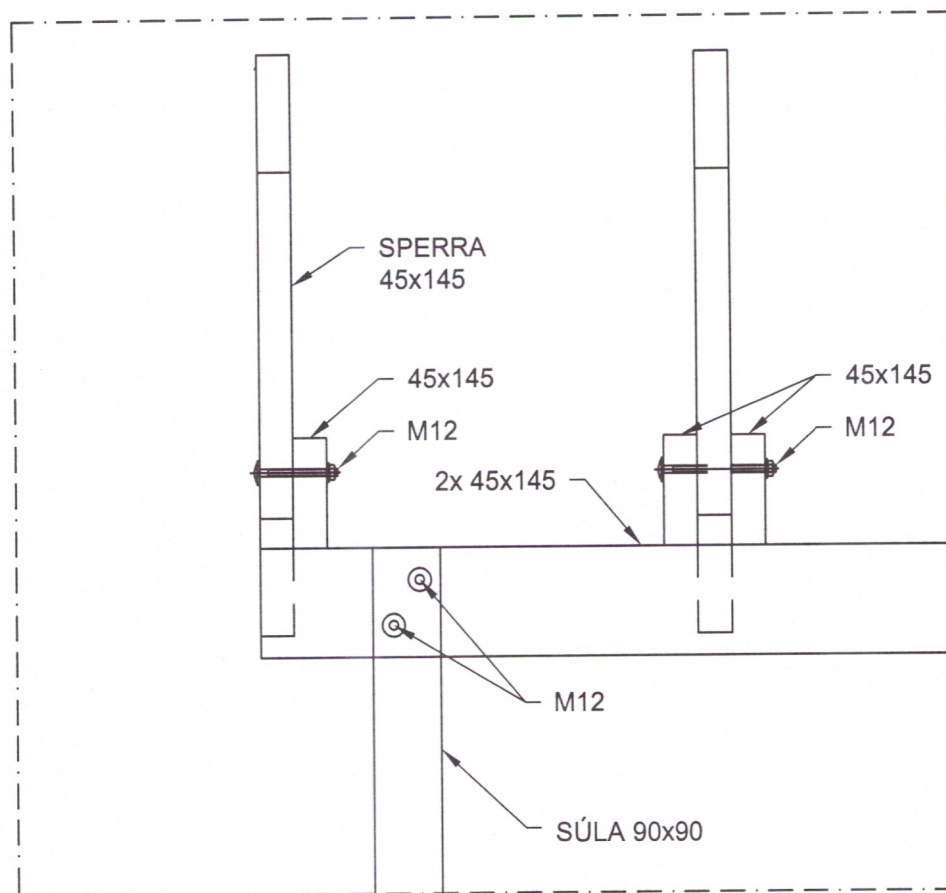
08 DEILI B005 1:10
