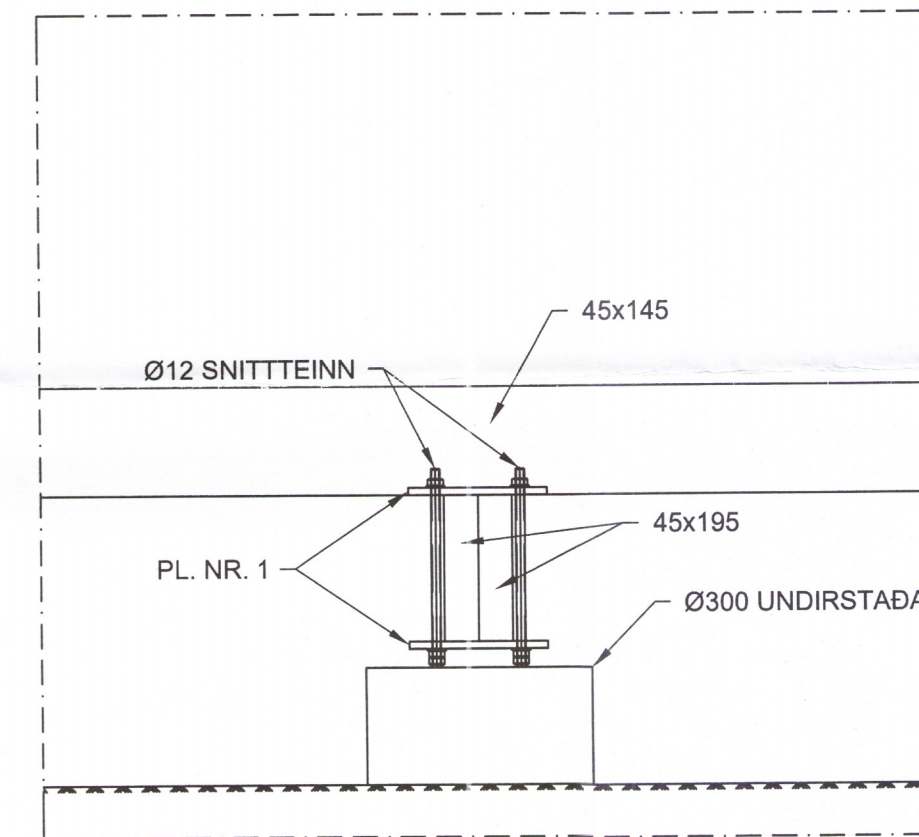
11 DEILI B005 1:10
