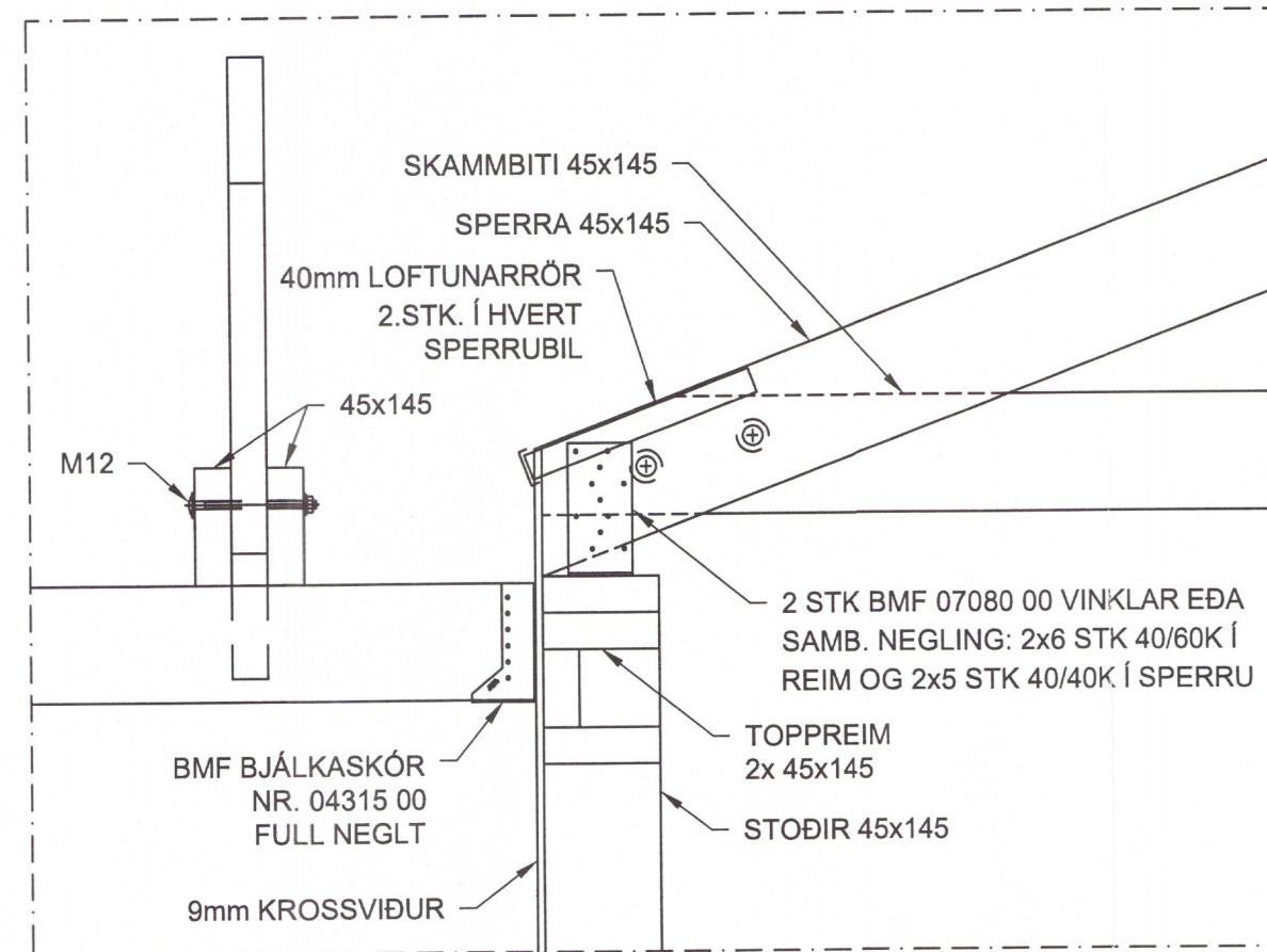
10 DEILI B005 1:10
