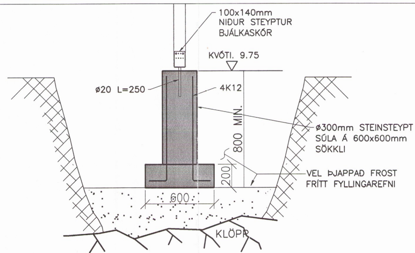
DEILI B SÚLA SCALE=1:20
