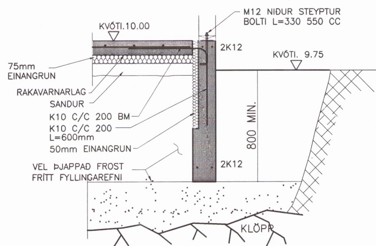
DEILI A SÖKKULL SCALE=1:20
