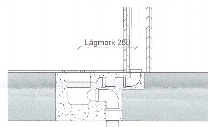
GÓLFNIÐURFALL MEÐ GEGNUMRENNSLI, MKV.:1:10
