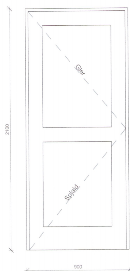
H1, 1 stk., hurð oppnast inn, til vinstri.
