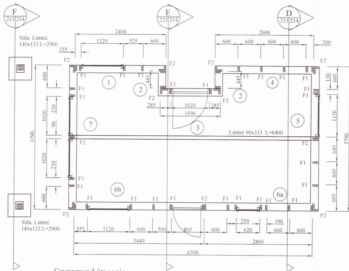
Grunnmynd útveggja MKV. 1:50
