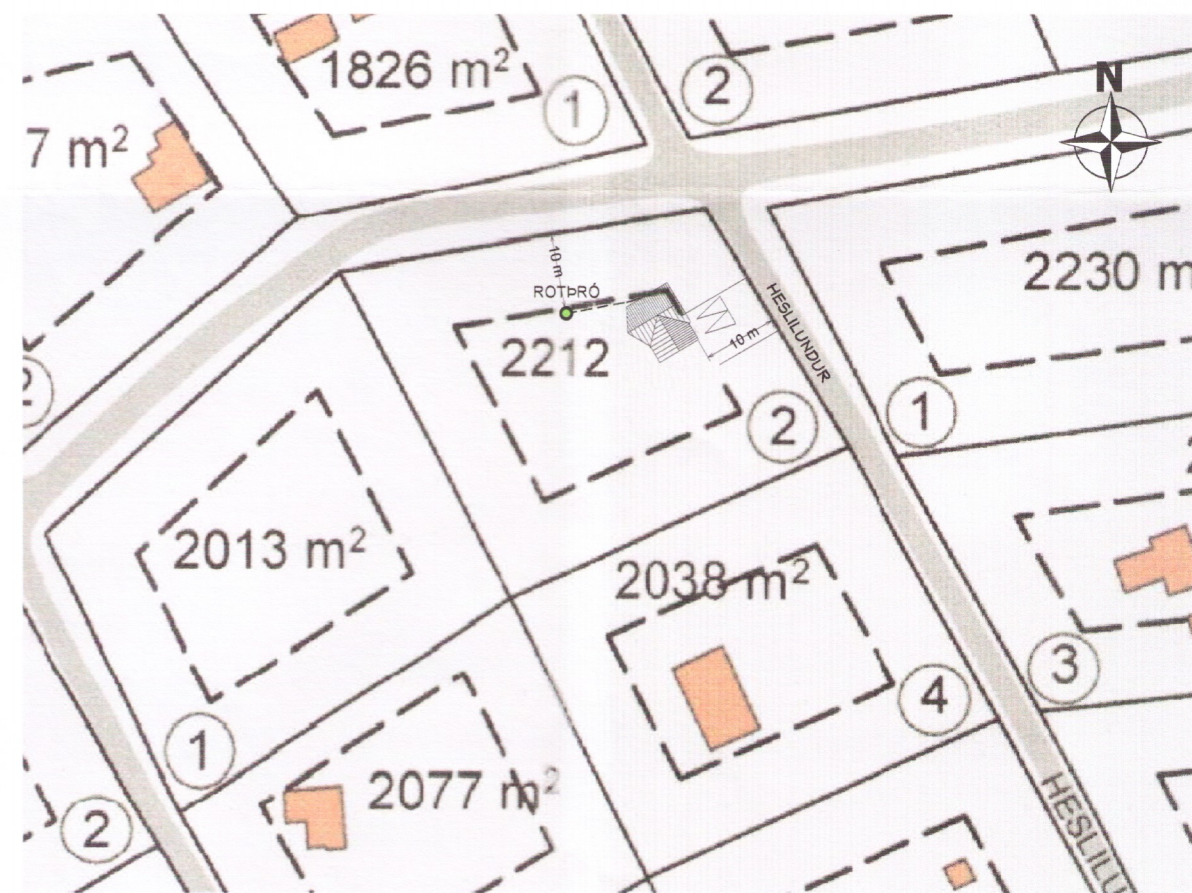
AFSTÖÐUMYND, 1:1000
