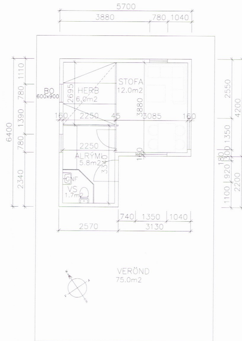
GRUNNMYND
