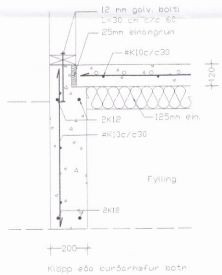
SNİÐ A-A útveggur sökkla
