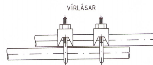
SAMTENGING STEYPUVEINA SETJA SKAL TVO VÍRLÁSA Á HVER SAMSEYTI
