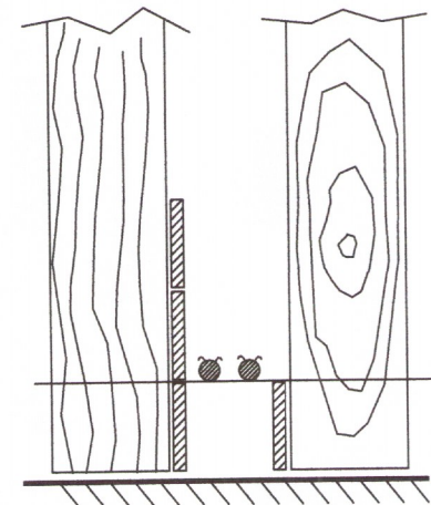
SNÍÐ A - A Í SÖKKULVEGG SÝND ERU 2 NEDSTU STEYPU- STYRKJARJÁRN Í STEYPU- MÖTI OFAN Á NEDSTU MÖTAVÍRUM
