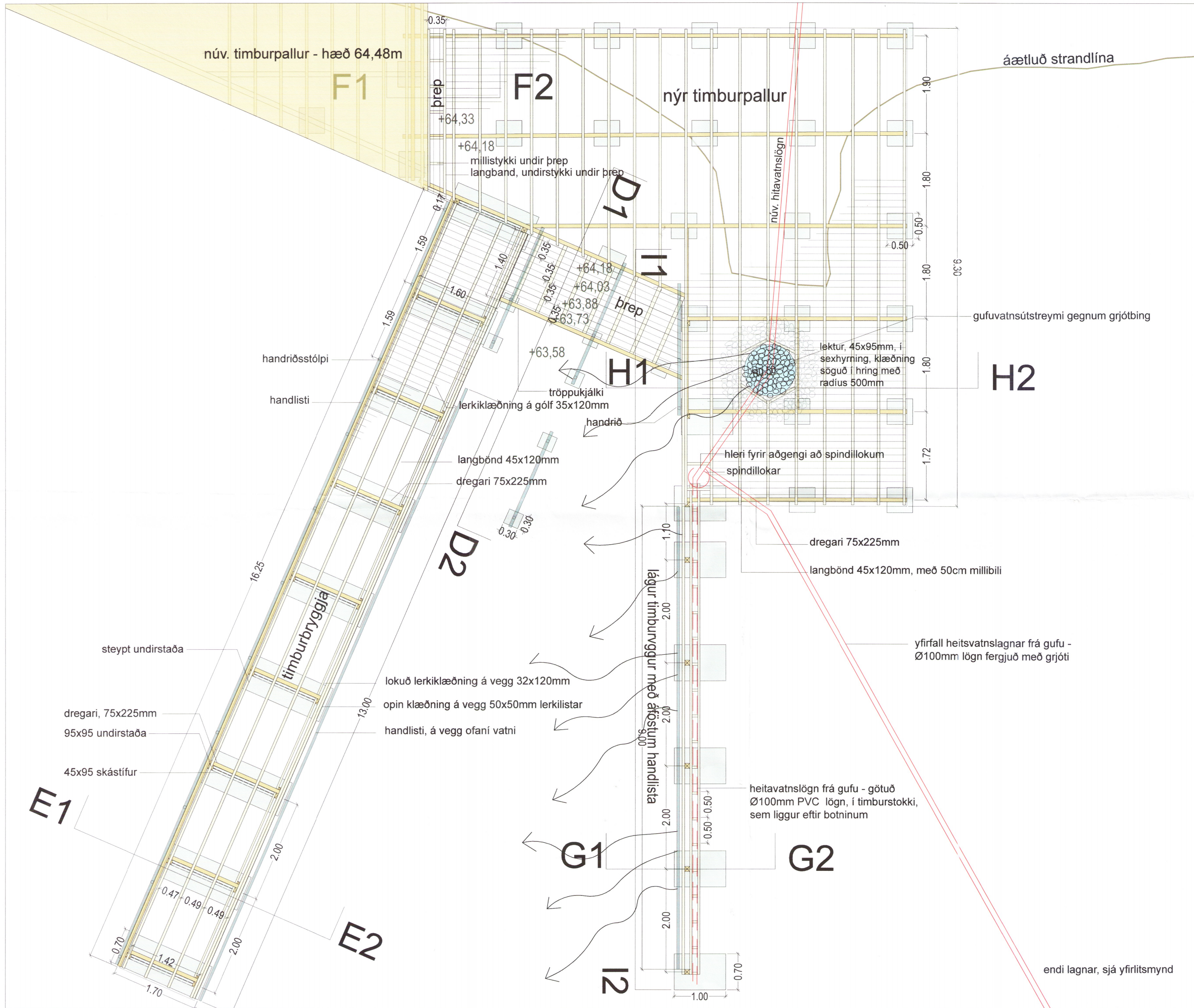
Grunnmynd bryggju og timburpalls, mkv. 1:50
