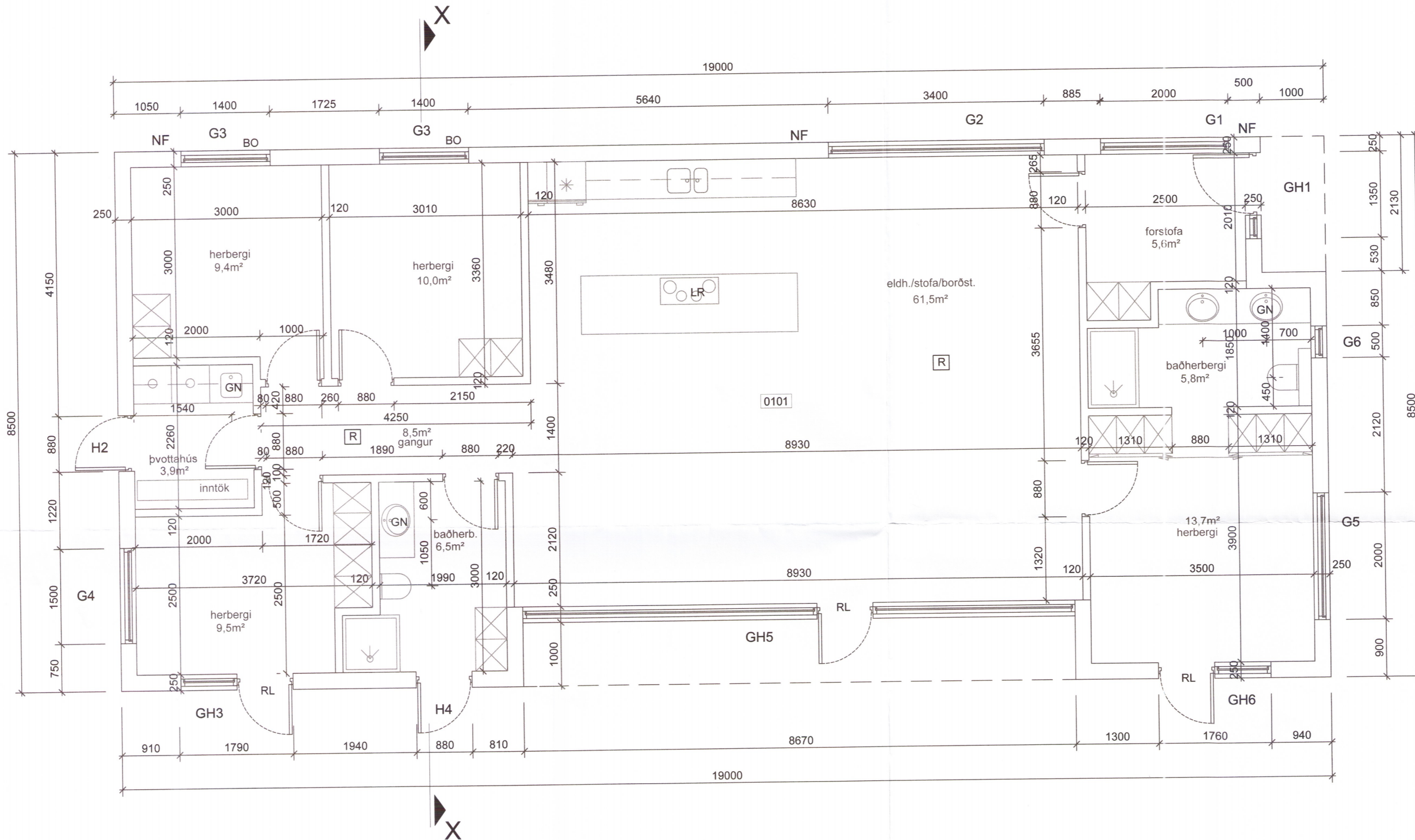
GRUNNMYND 1:50
