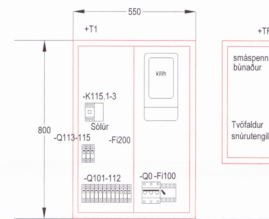
Töfluútlit - M 1:10
