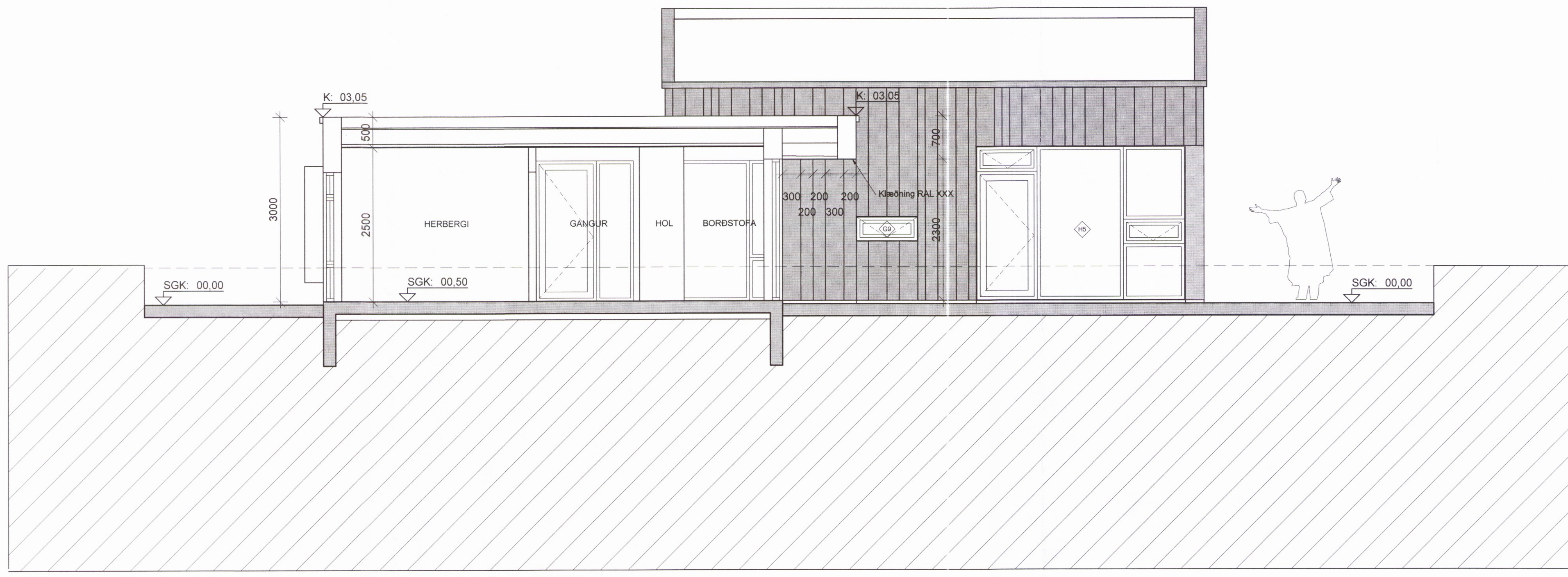
SNEIÐING C-C 1:50
