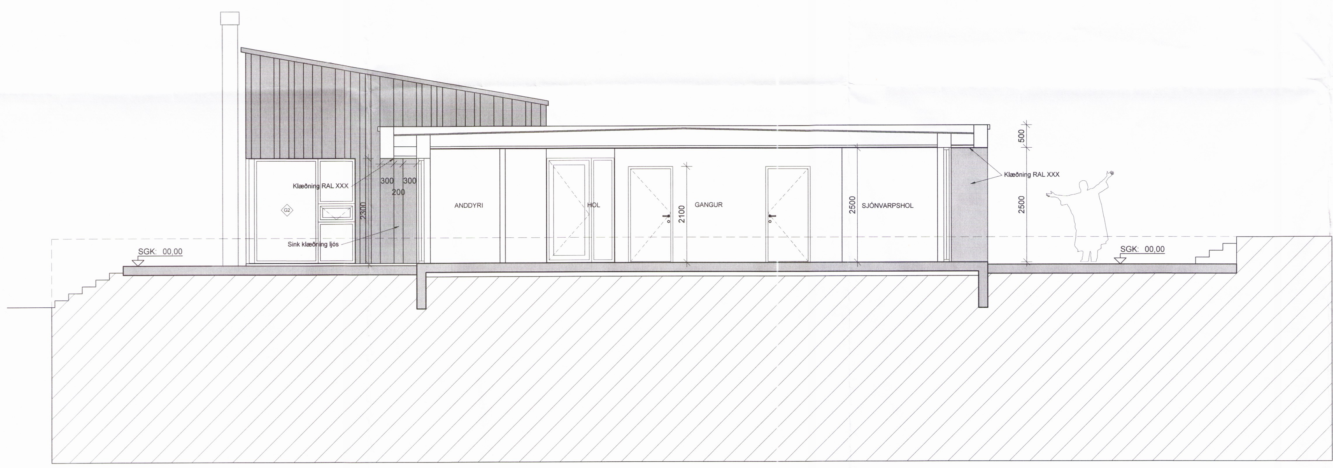
SNEIÐING D-D 1:50
