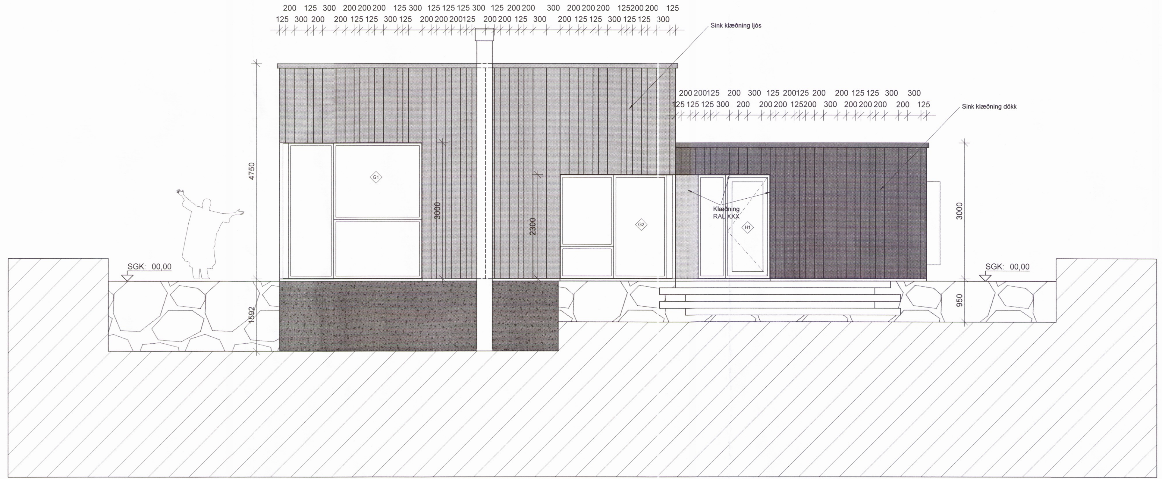
ÚTLIT SUÐVESTUR 1:50
