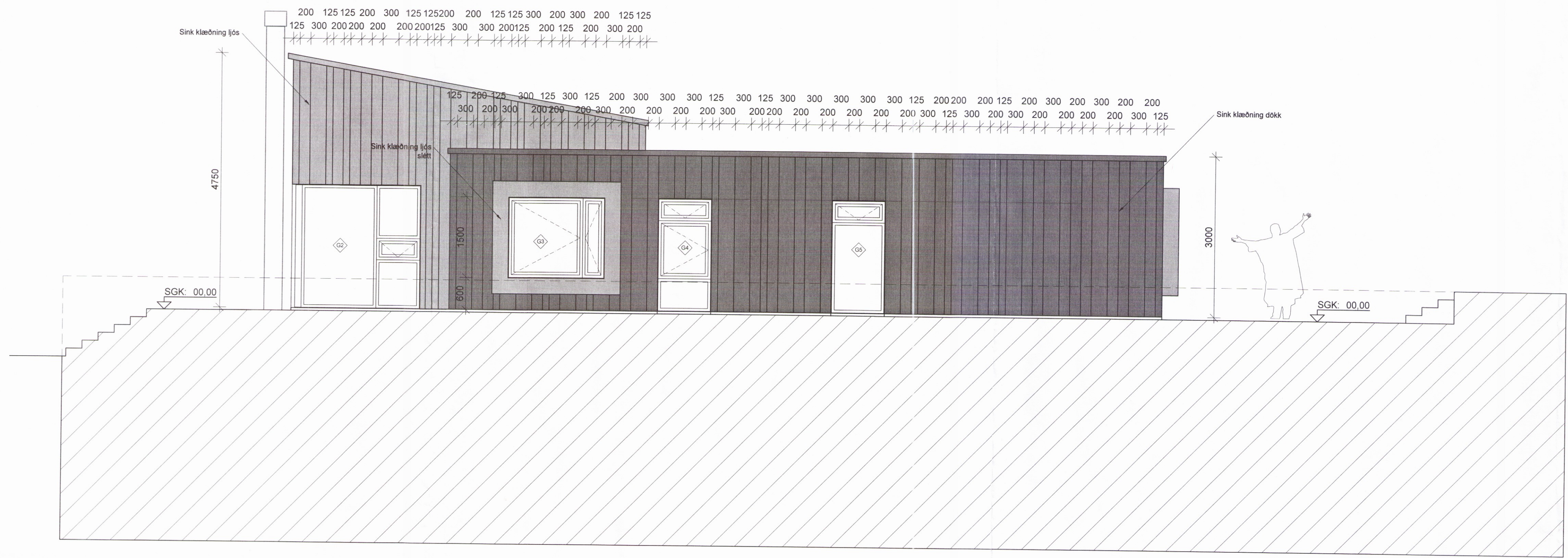
ÚTLIT SUDAUSTUR 1:50
