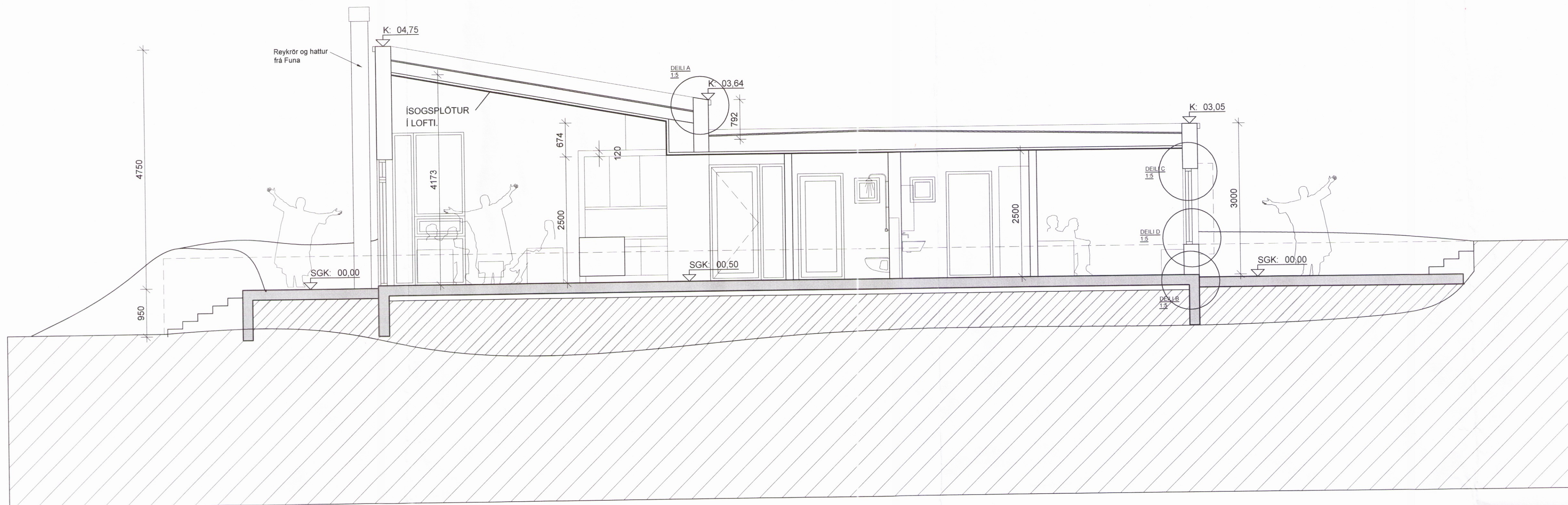
SNEIÐING A-A 1:50
