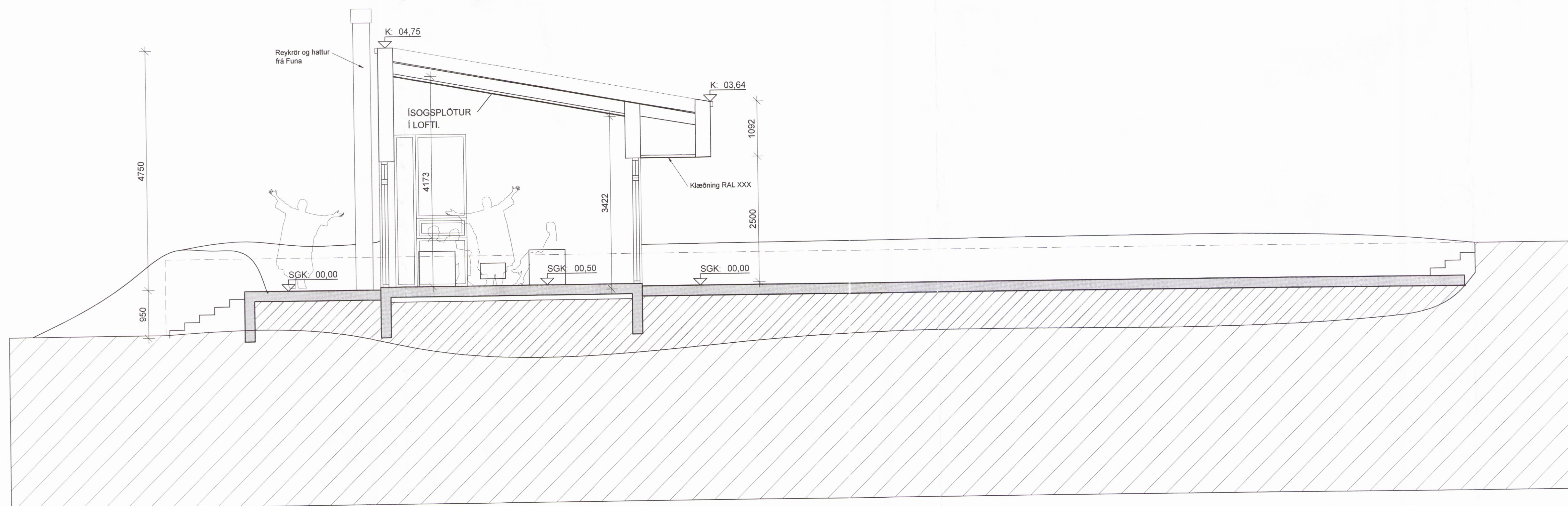
SNEIÐING B-B 1:50
