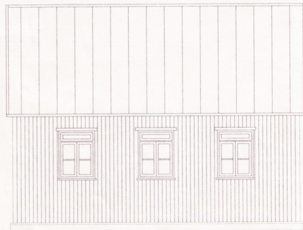
SUÐUR / NORÐUR, 1:50
