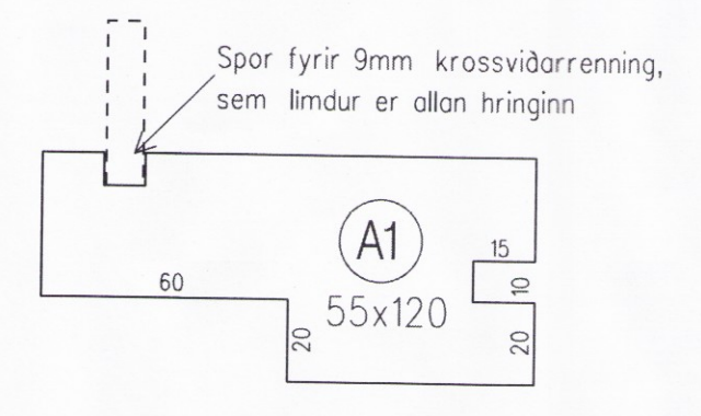
Gluggasnið - 1:2
