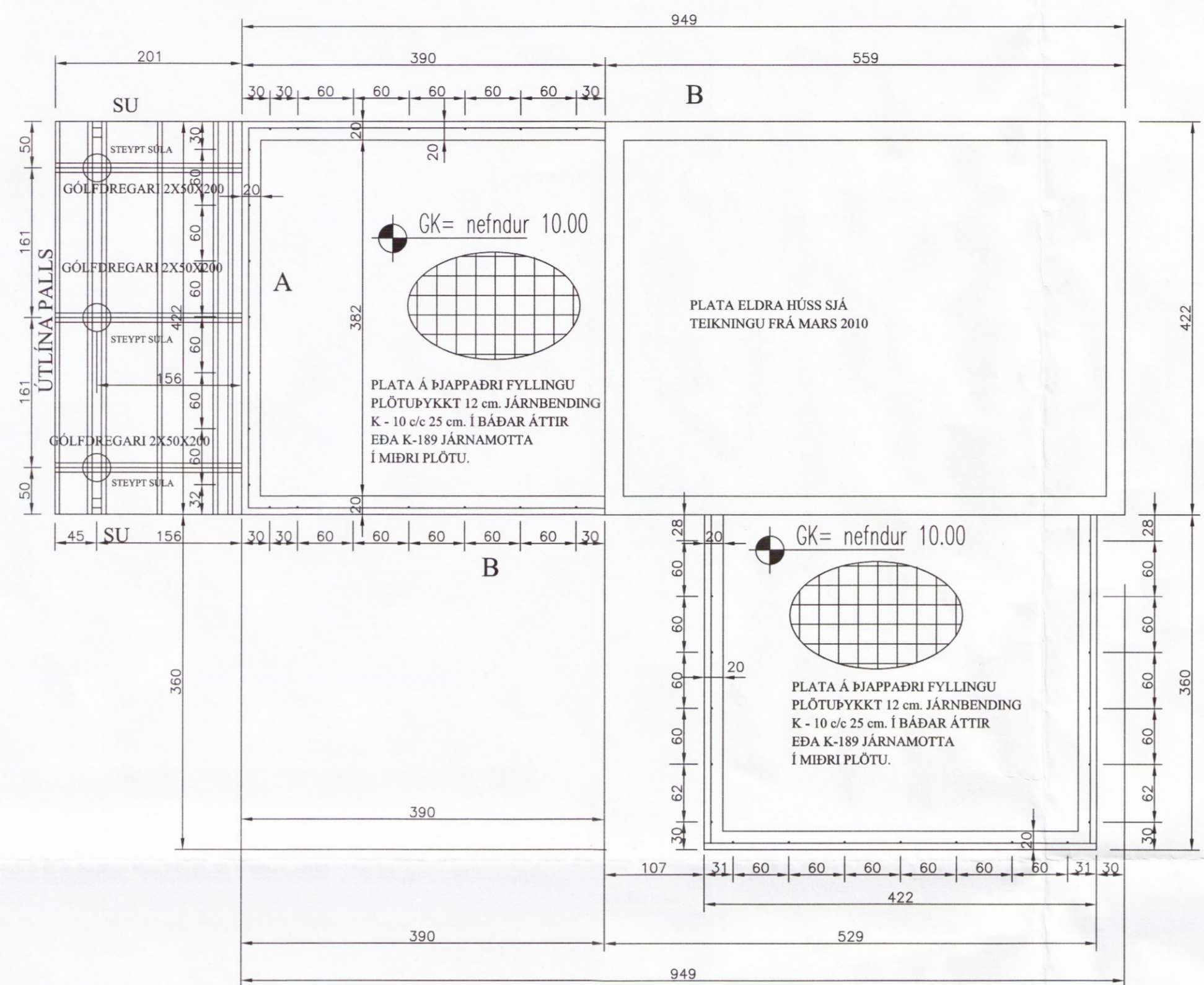
Grunnmynd sökkjar, 1:50
