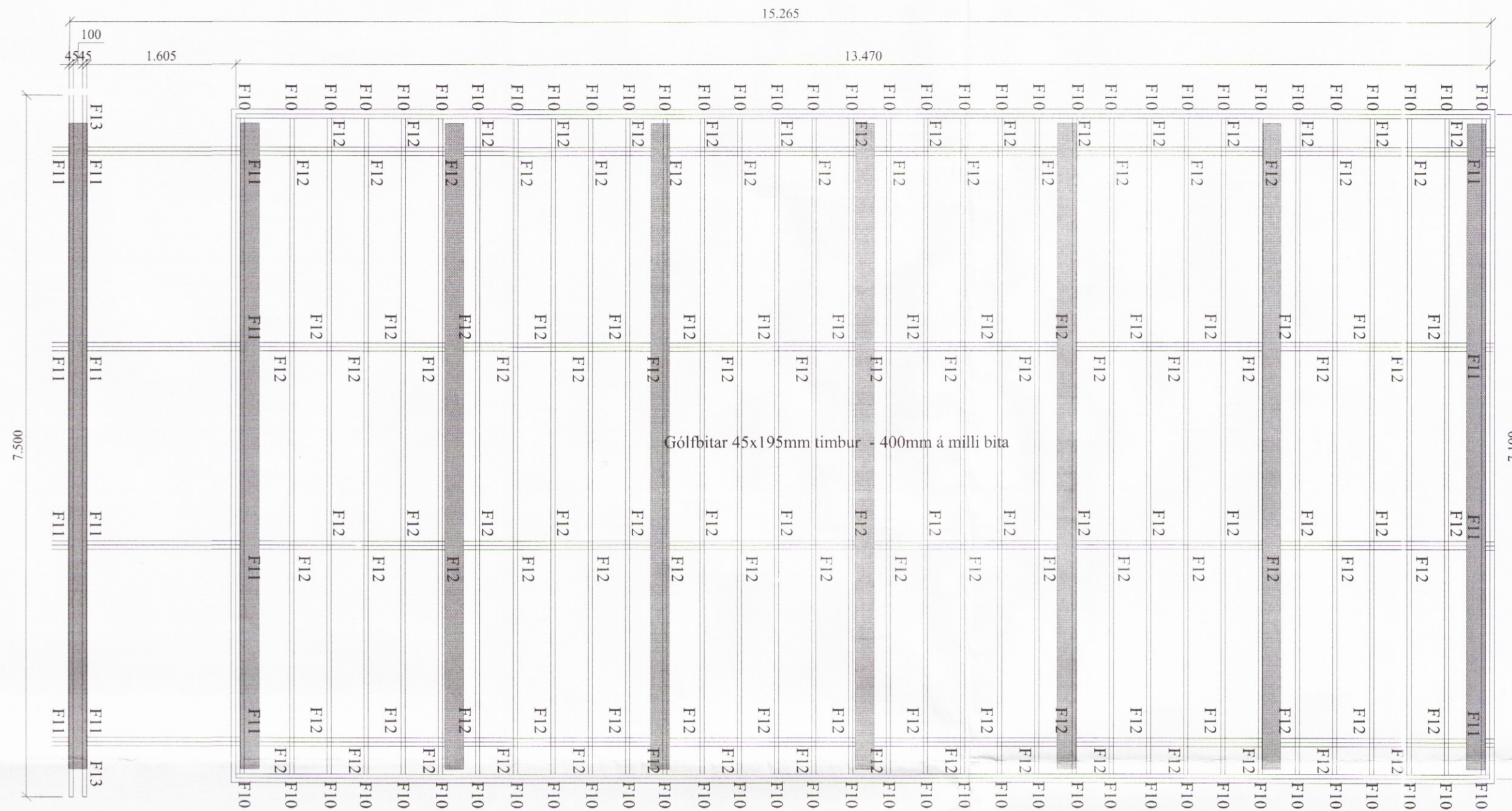
Grunmynd gólfbita mkv. 1:50
