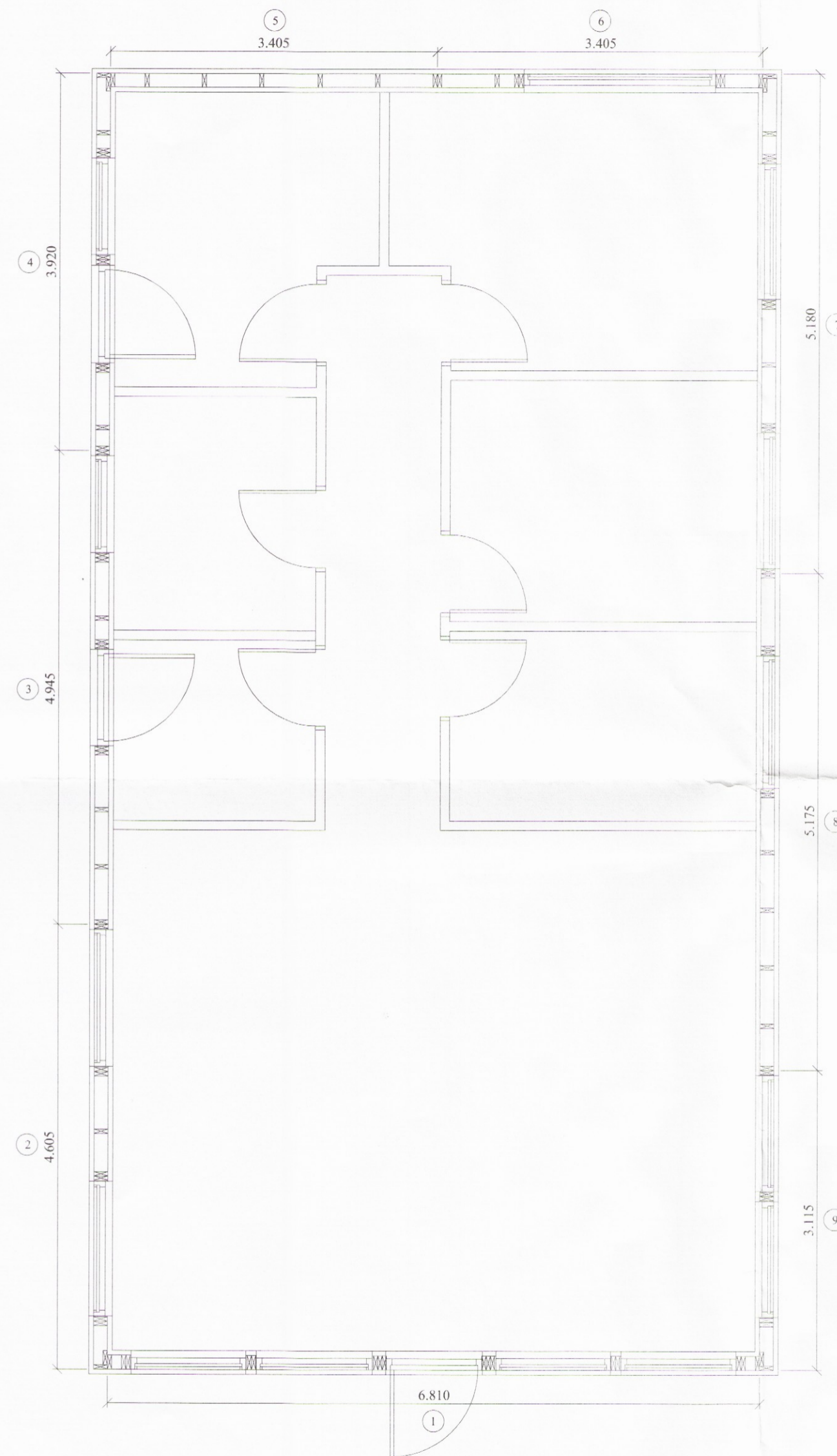
Grunnmynd grindur mkv. 1:50
