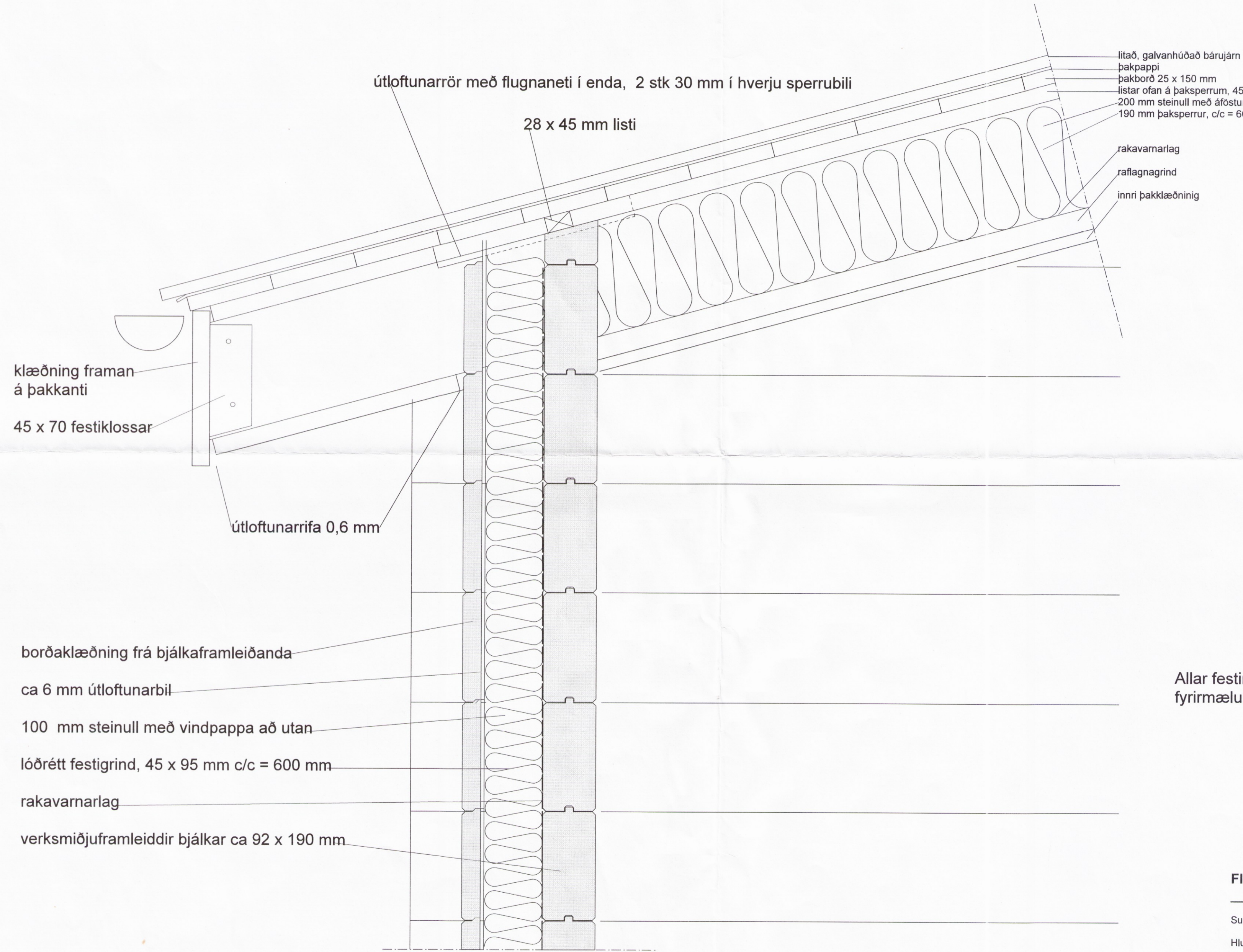
Sneiðing í útvegg, þak og þakkant, mkv. 1:5
