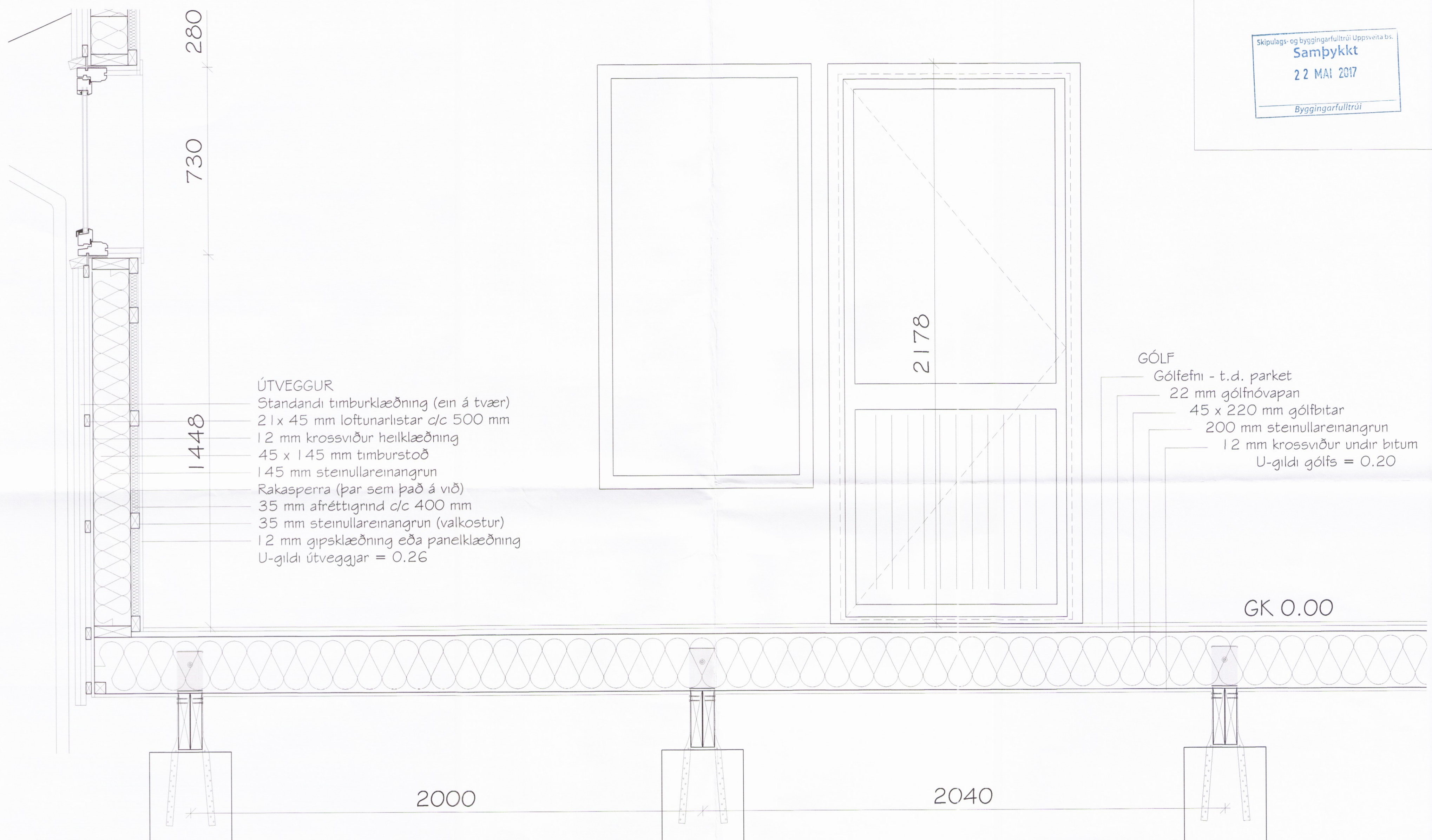
Deiliteikning B
