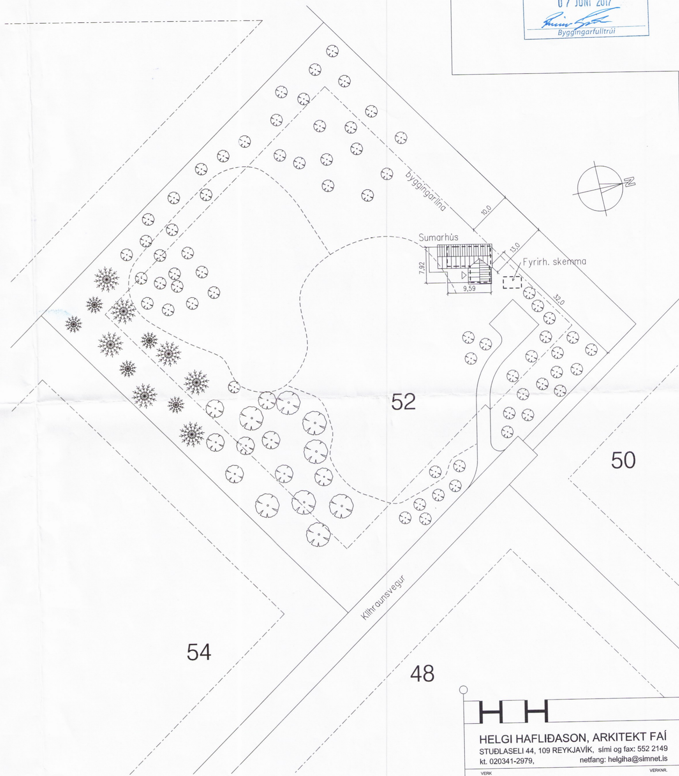
Afstöðumynd 1:500
