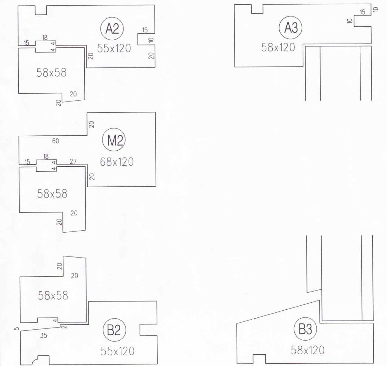
Gluggasnið - 1:2
