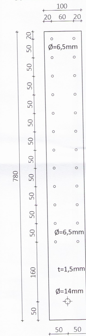
Stálfesting F1 Mkv. 1:5
