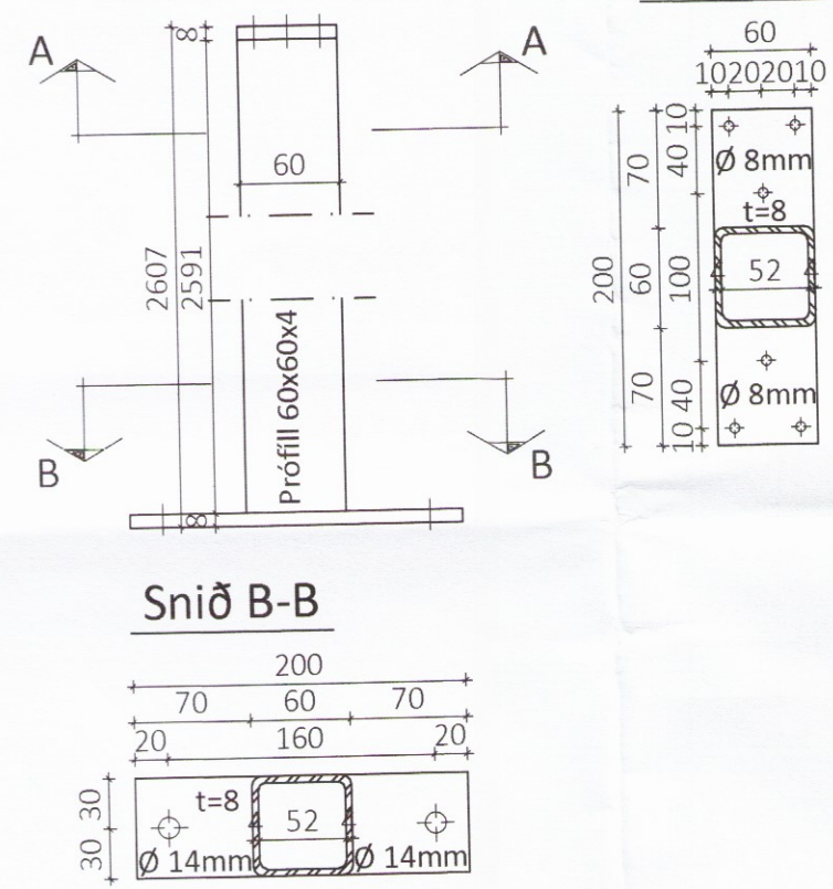
Stálsúla SU1 Mkv. 1:5 Samtals 4 stk
