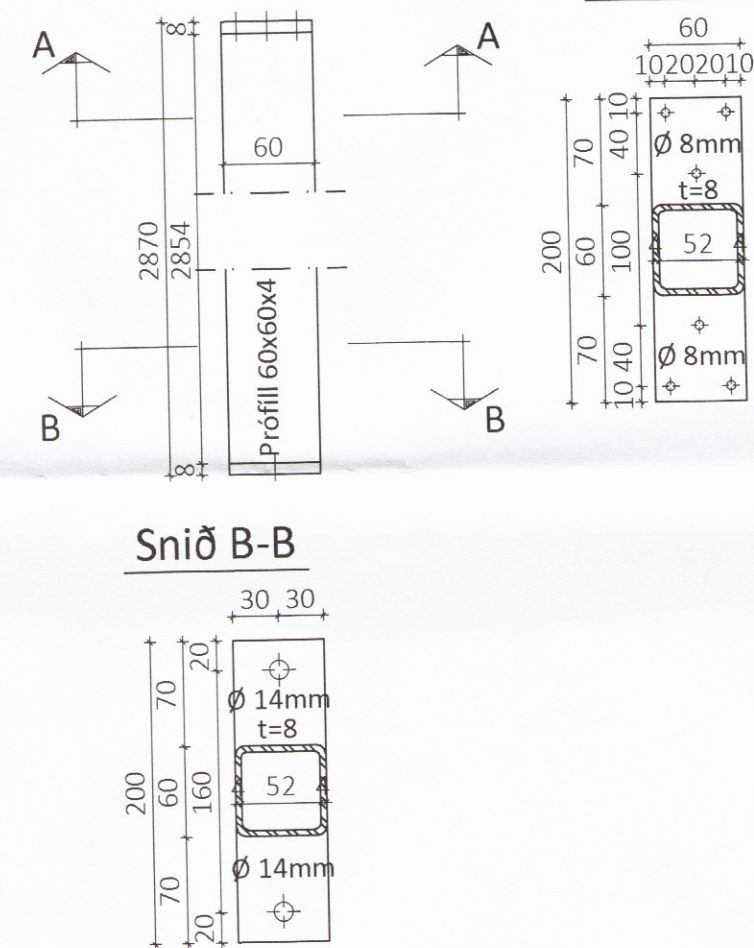
Stálsúla SU2 Mkv. 1:5 Samtals 4 stk
