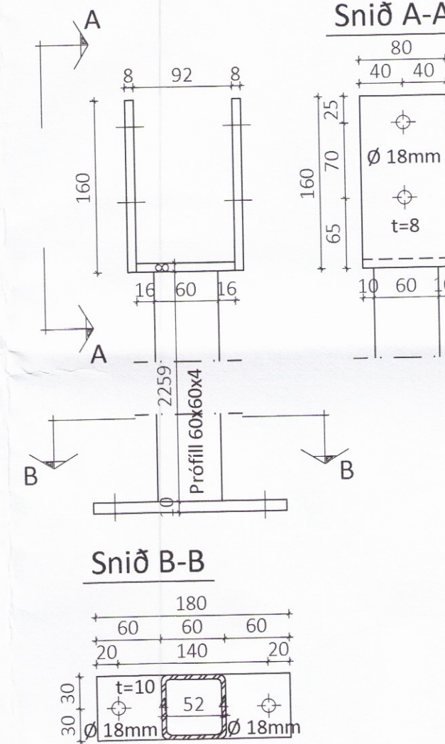
Stálsúla SU3 Mkv. 1:5 Samtals 2 stk
