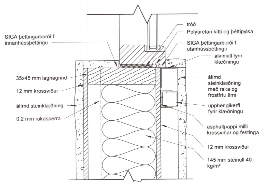
6 frág. glugga við steinklæðningu 1 : 5
