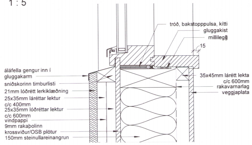
2 frágangur neðan við glugga 1 : 5
