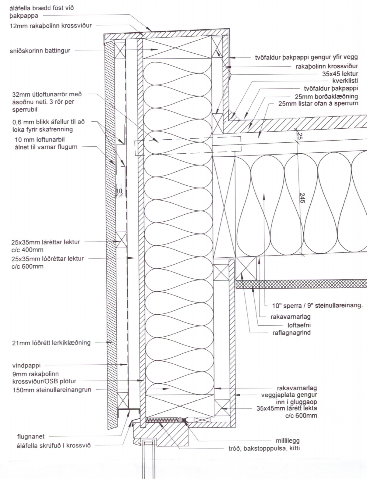
1 frág. ofan við glugga / vegg og þak 1 : 5
