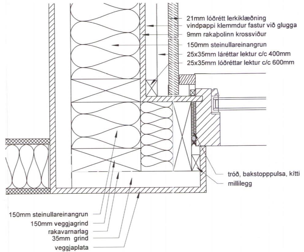
5 frág. við glugga/kverk í anddyri 1 : 5
