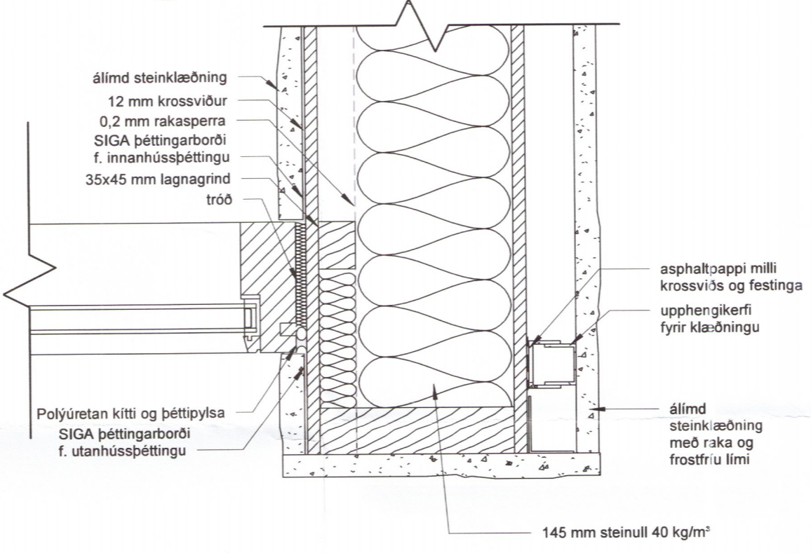
6 frág. glugga við steinklæðningu 1 : 5
