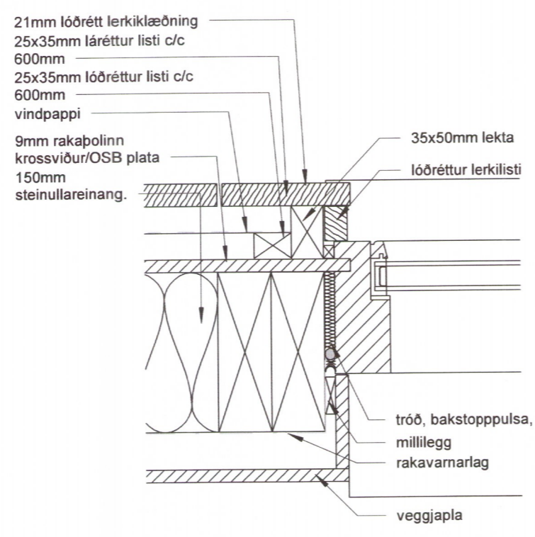
4 frág. við glugga - lárétt snið 1 : 5
