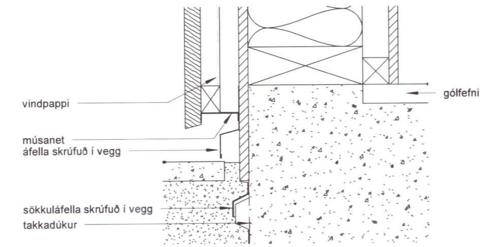
3 frágangur við sökkul 1 : 5
