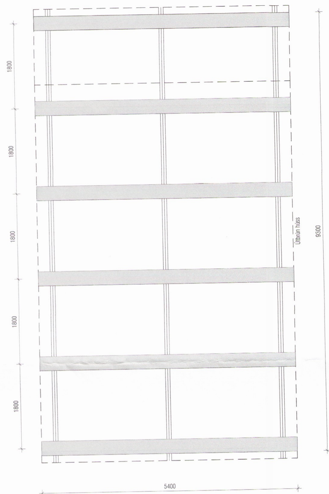
UNDIRSTÖÐUR - GRUNNMYND 1:50
