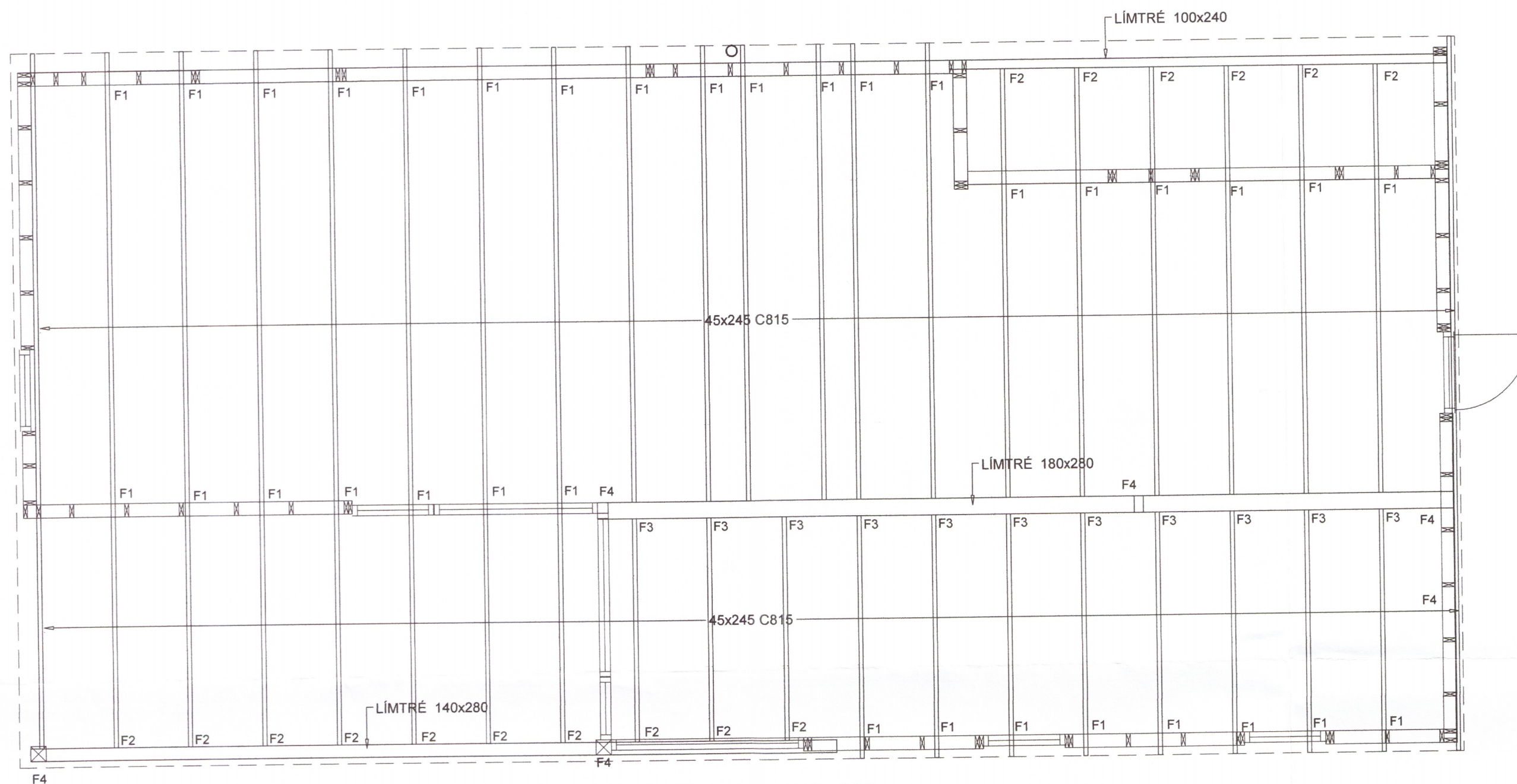
GRUNNMYND ÞAKS, 1:50
