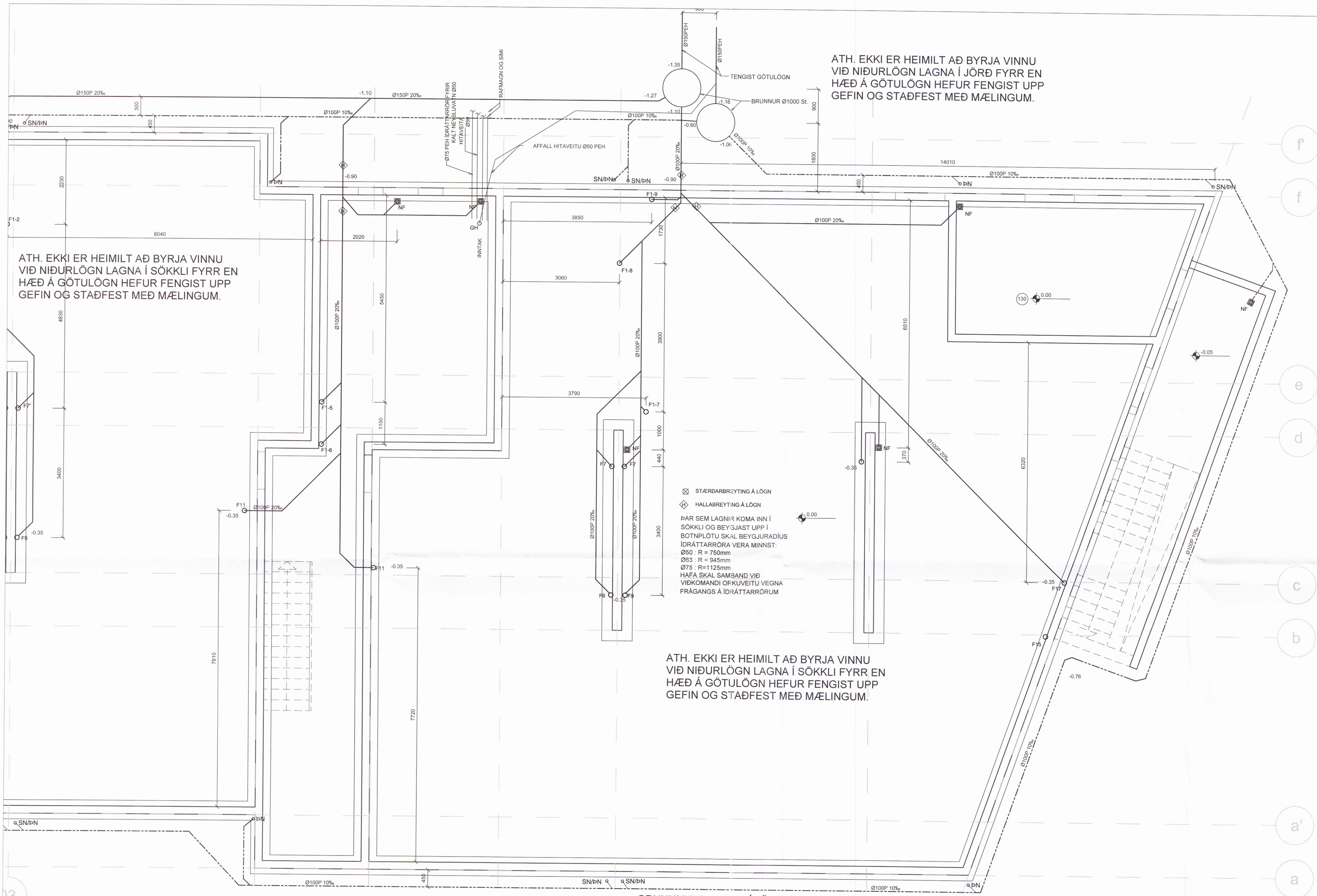
GRUNNMYND LAGNA Í JÖRÐ 1:50
