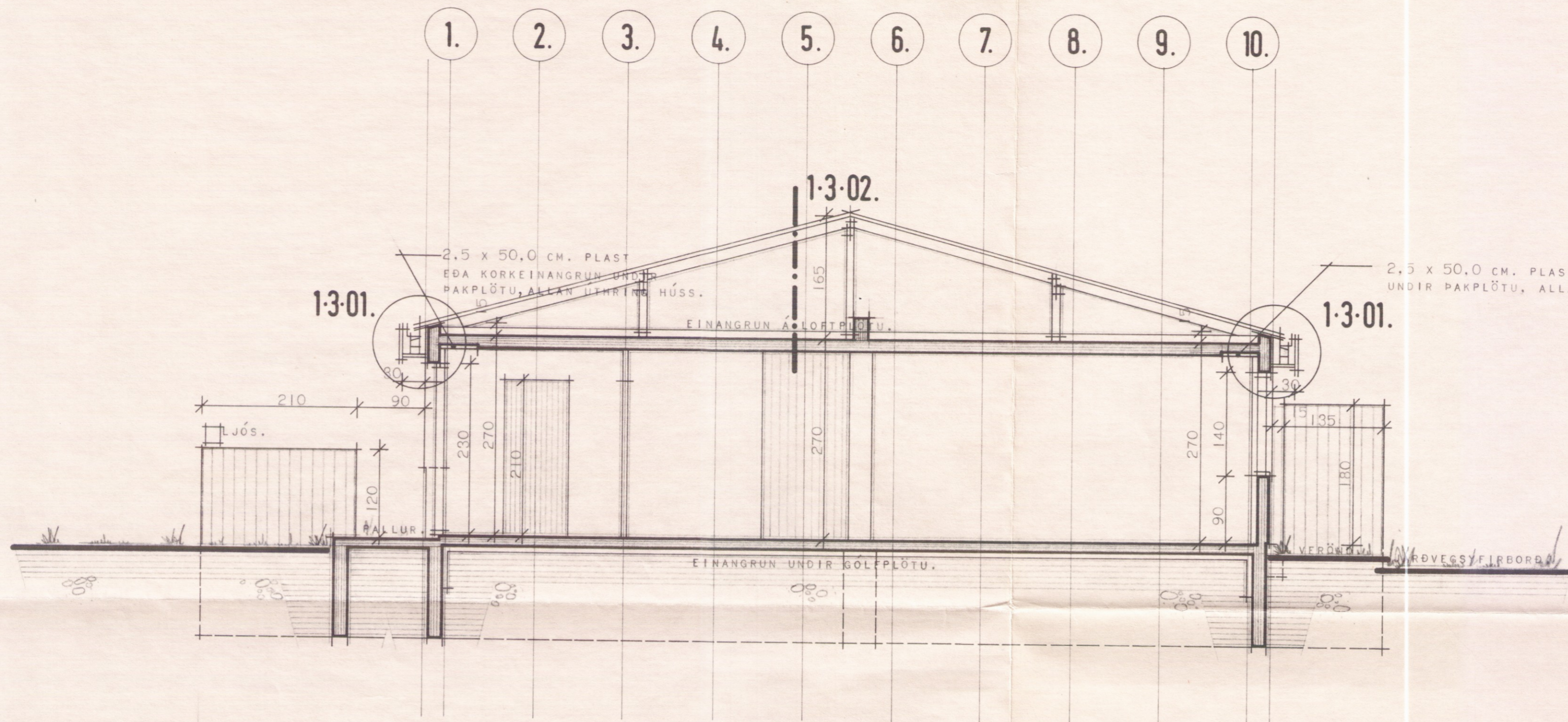
ÞVERSNEIÐING A - A.
