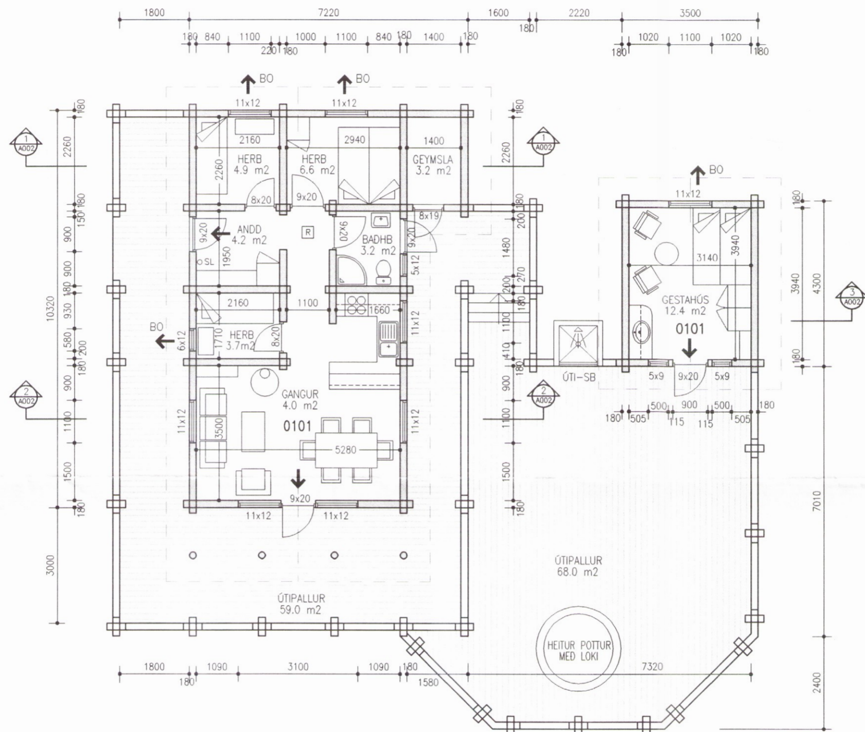
GRUNNMYND 1:100
