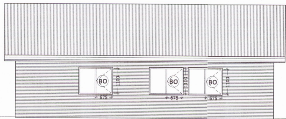
Útlit norður 1:100
