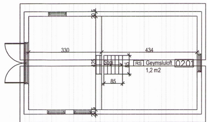
Grunnmynd geymsluloft kvarði 1:100
