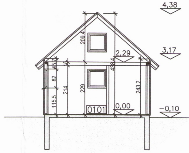
Snið A kvarði 1:100
