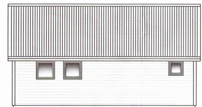
Útlit Austur kvarði 1:100
