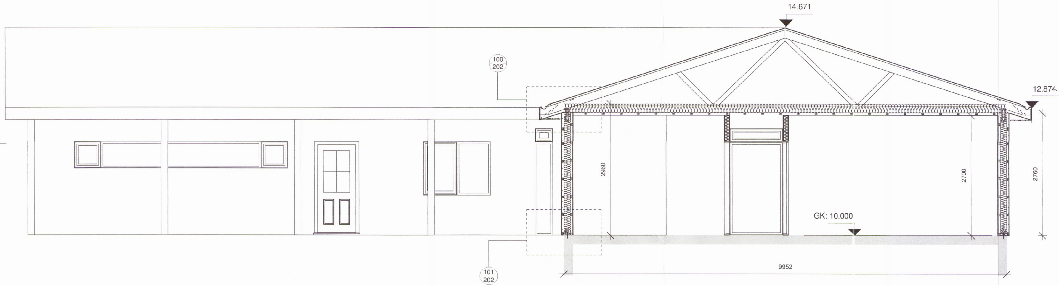
Snið A-A 1 : 50
