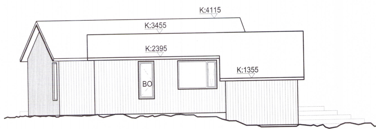
5 ÚTLIT AUSTUR 1:100
