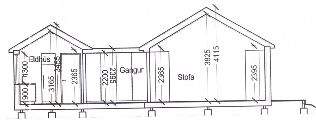
3 SNID 1:100
