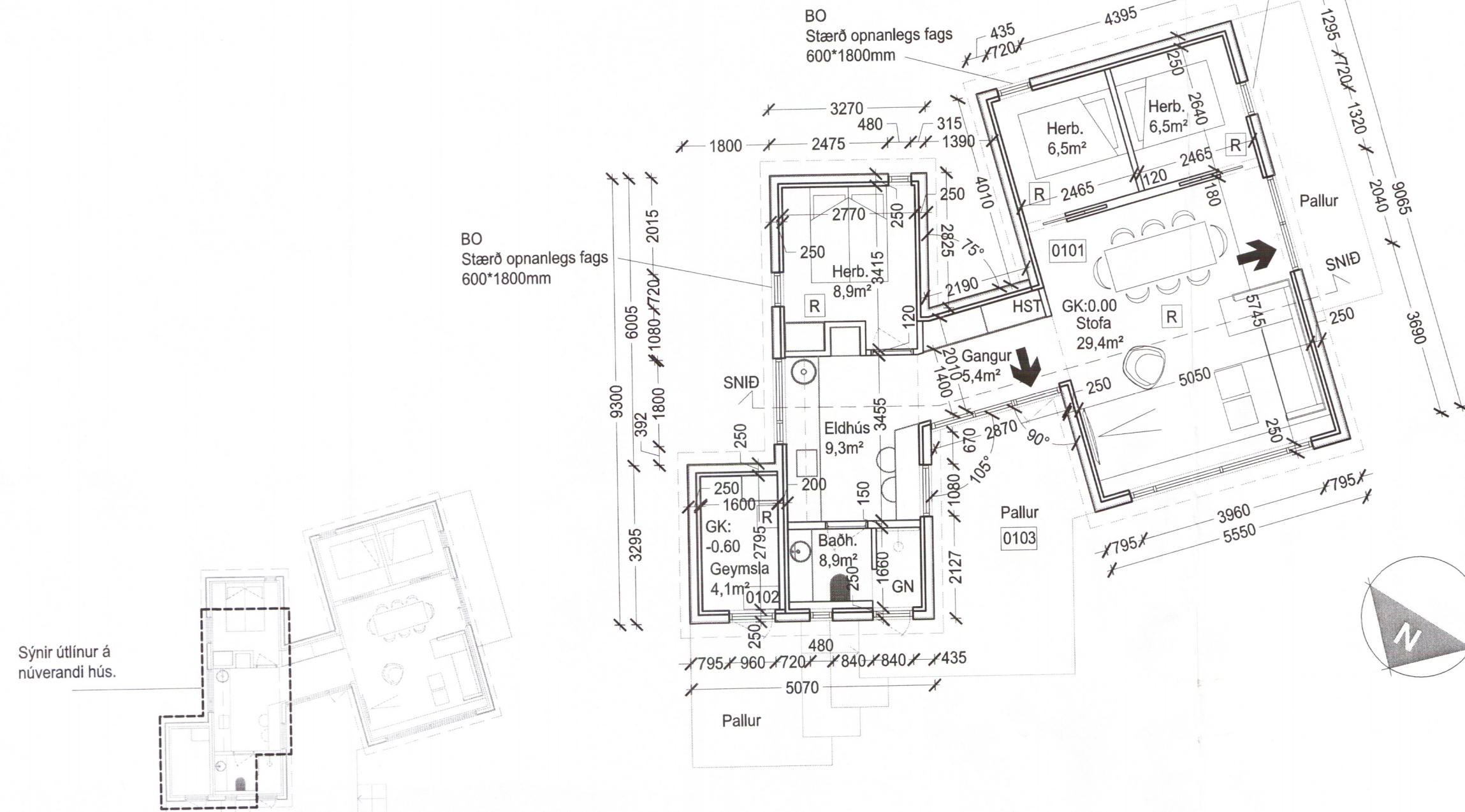
1 YFIRLITSMYND 1:200
