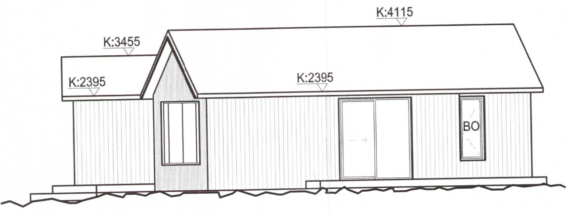
7 ÚTLIT AUSTUR 1:100
