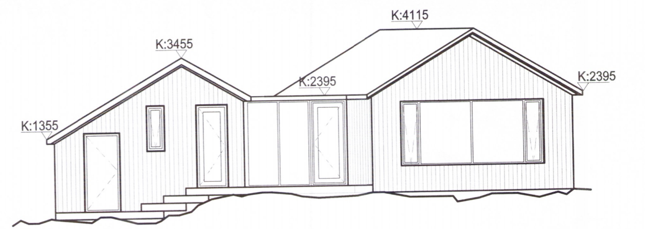
4 ÚTLIT NORÐUR 1:100
