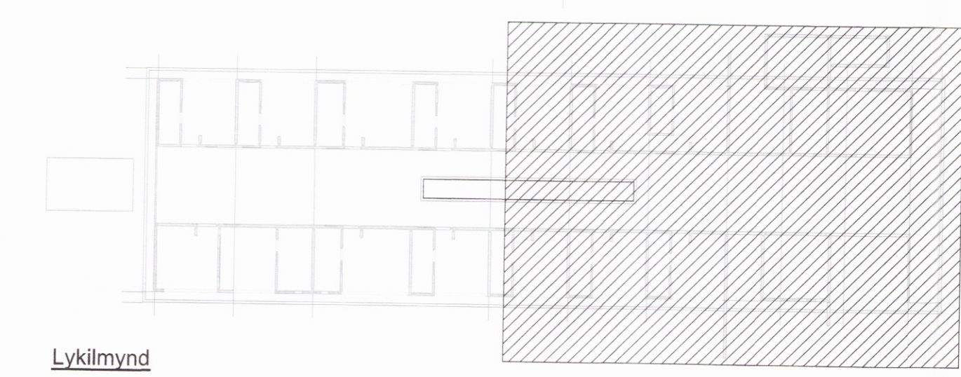
Grunnmynd 1. hæðar, veggeiningar 1:50
