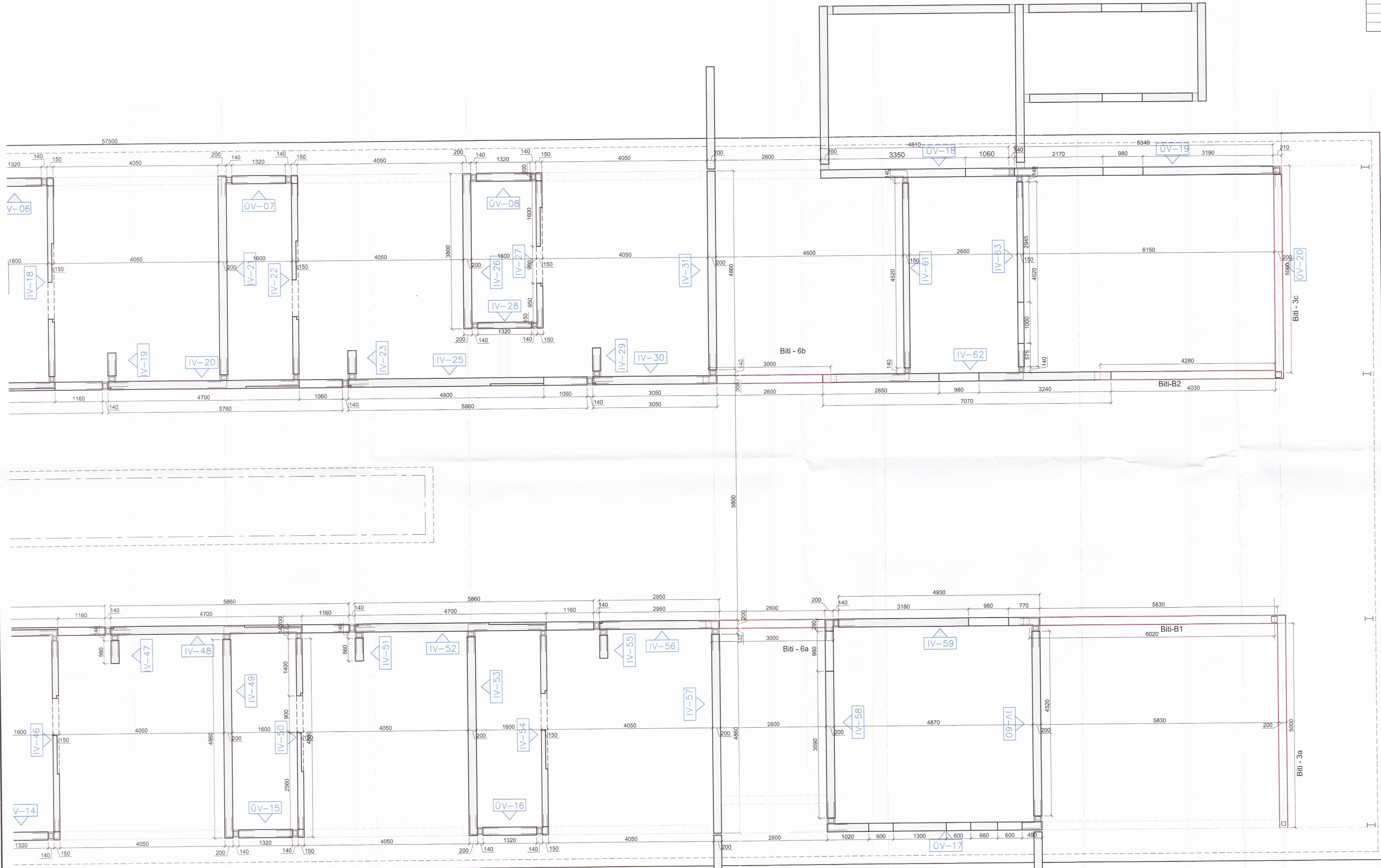
Grunnmynd 1. hæðar, veggeiningar 1:50
