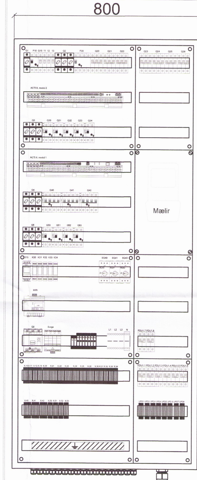
Útlit töflu kvarði 1:8 Sjá stærri mynd á teikningu R-06
